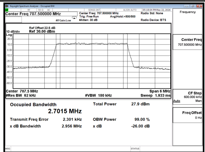
OCC B12 3M CH23095 256QAM
