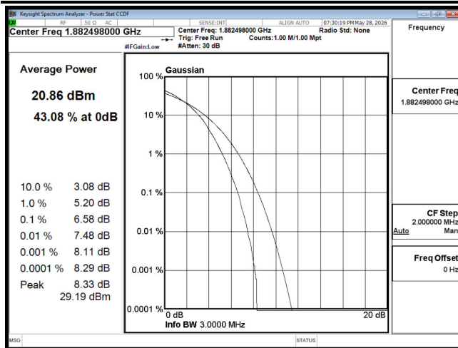
PTAR B25 3M CH26365 64QAM
