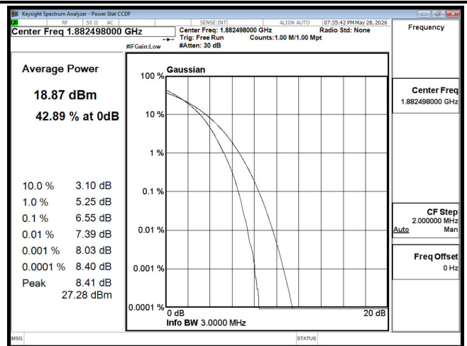
PTAR B25 3M CH26365 256QAM
