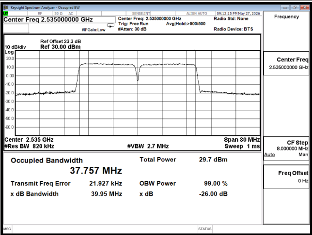
OCC B7 20M CH21001(100,0),20M CH21199(100,0) QPSK
