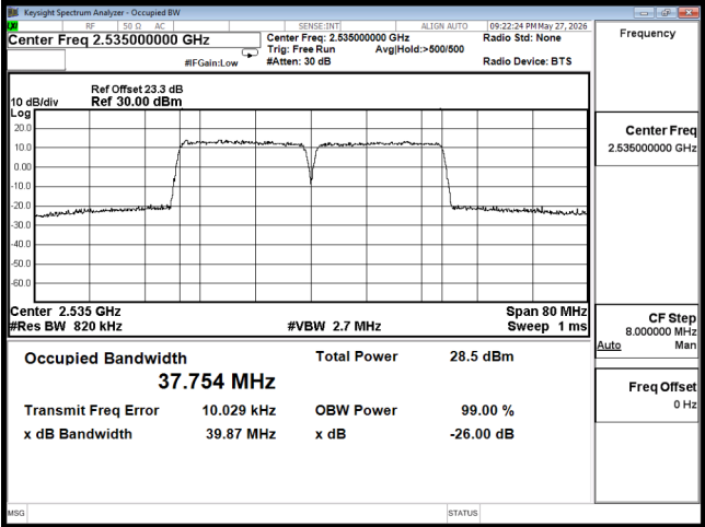
OCC B7 20M CH21001(100,0),20M CH21199(100,0) 64QAM
