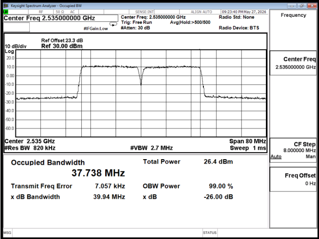
OCC B7 20M CH21001(100,0),20M CH21199(100,0) 256QAM
