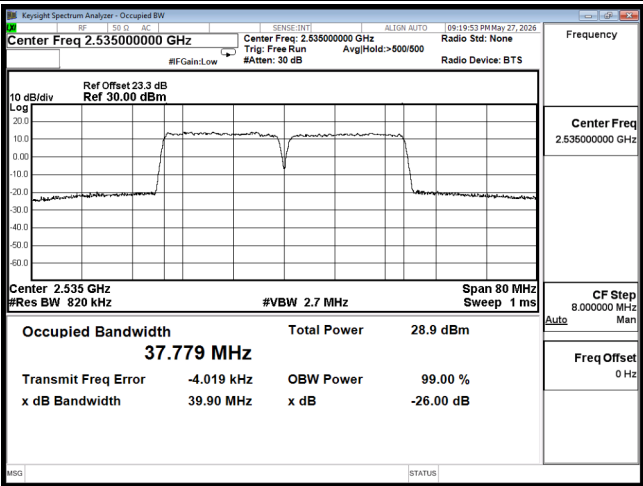
OCC B7 20M CH21001(100,0),20M CH21199(100,0) 16QAM
