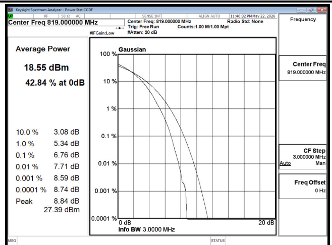
PTAR B26 3M CH26740 256QAM
