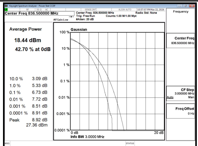
PTAR B26 3M CH26915 256QAM
