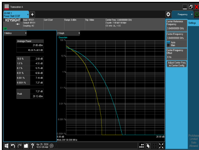
PTAR n77 60M CH656000 QPSK
