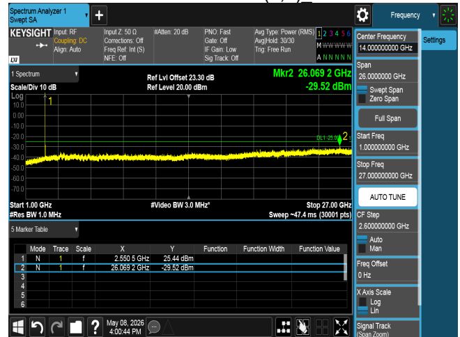
CSE n7 20M CH512000 BPSK(1,1)_
