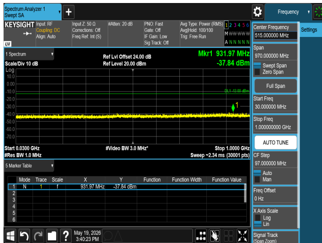
CSE n77 30M CH631000 BPSK(1,1)
