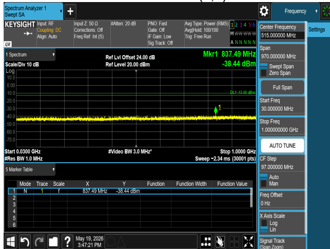
CSE n77 60M CH633334 BPSK(1,1)
