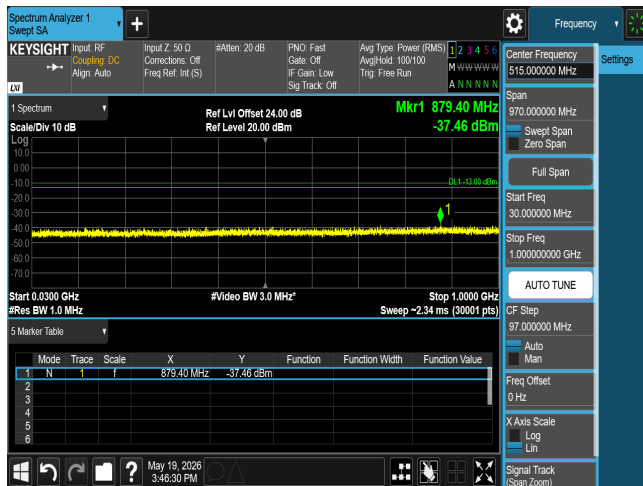
CSE n77 60M CH632000 BPSK(1,1)
