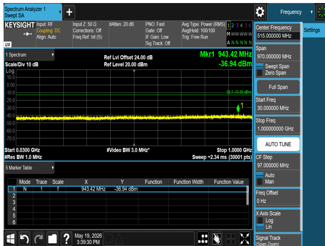
CSE n77 25M CH630834 BPSK(1,1)
