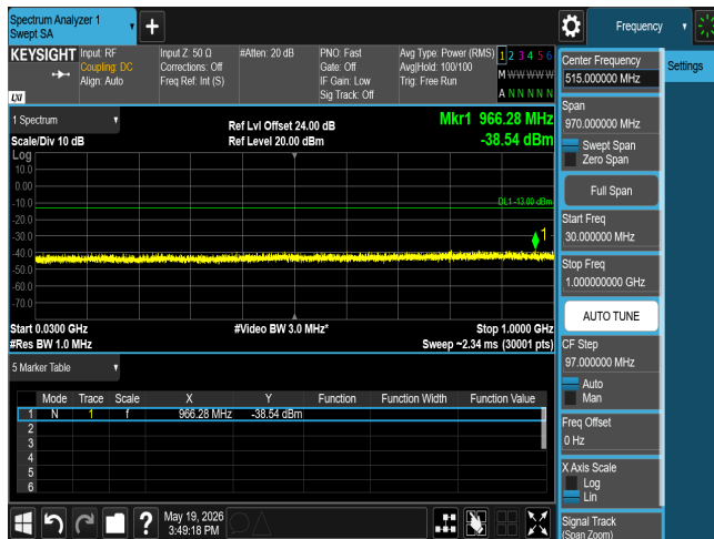
CSE n77 70M CH632334 BPSK(1,1)
