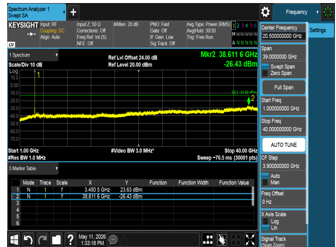
CSE n77 40M CH631334 BPSK(1,1)
