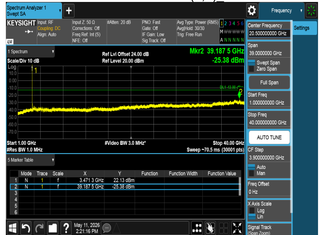
CSE n77 60M CH633334 BPSK(1,1)
