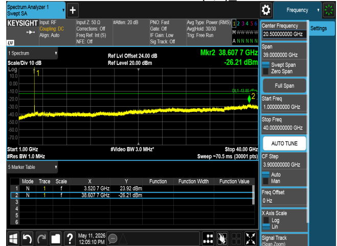
CSE n77 30M CH635666 BPSK(1,1)_
