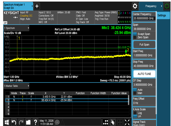
CSE n77 25M CH630834 BPSK(1,1)
