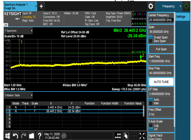
CSE n77 15M CH633334 BPSK(1,1)
