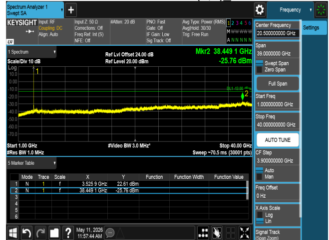
CSE n77 25M CH635832 BPSK(1,1)_
