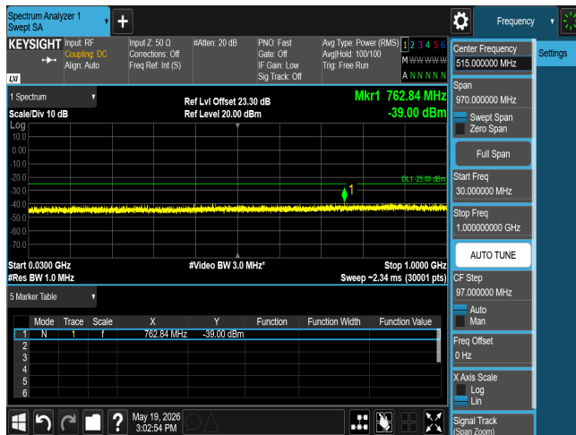
CSE n41 90M CH508200 BPSK(1,1)
