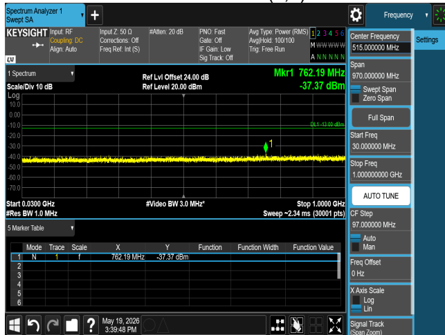
CSE n77 25M CH633334 BPSK(1,1)
