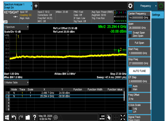
CSE n41 100M CH509202 BPSK(1,1)
