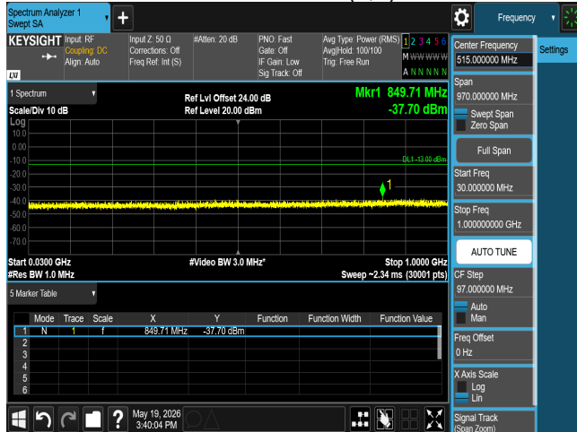
CSE n77 25M CH635832 BPSK(1,1)
