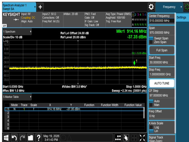
CSE n77 40M CH631334 BPSK(1,1)
