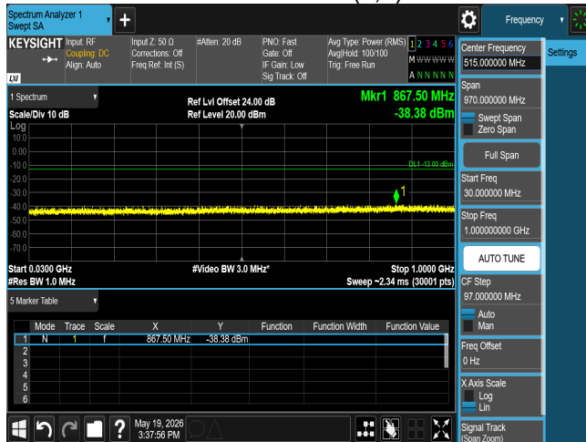
CSE n77 15M CH633334 BPSK(1,1)
