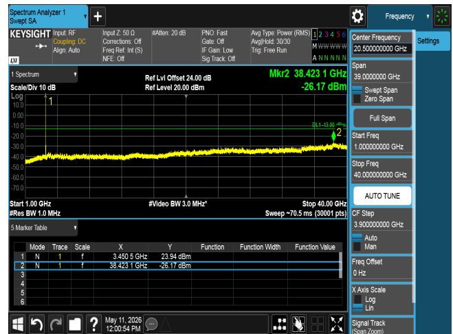
CSE n77 30M CH631000 BPSK(1,1)
