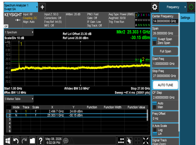
CSE n41 90M CH508200 BPSK(1,1)
