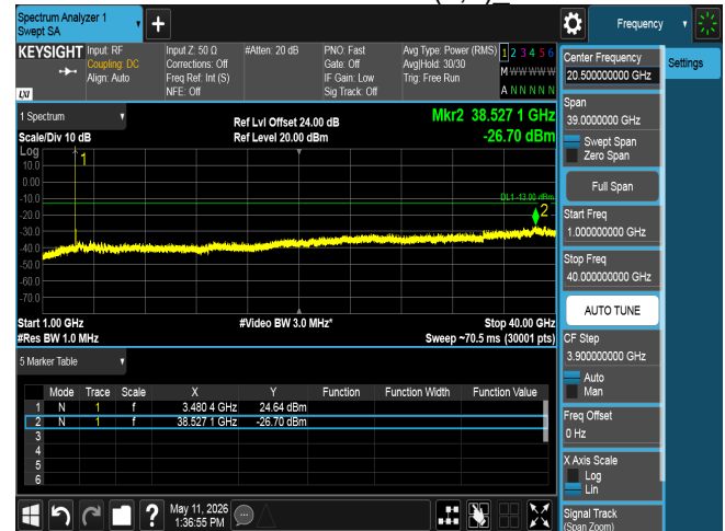
CSE n77 40M CH633334 BPSK(1,1)
