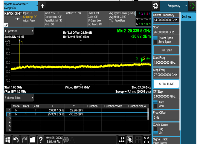
CSE n41 90M CH528996 BPSK(1,1)_
