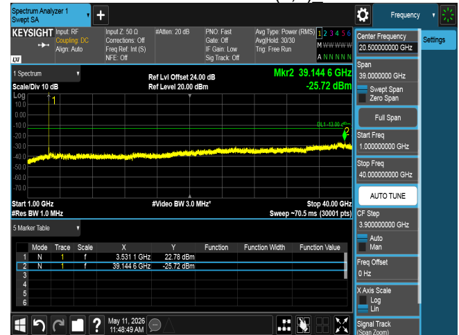
CSE n77 20M CH636000 BPSK(1,1)_
