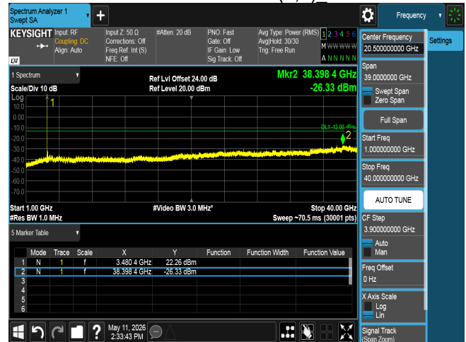
CSE n77 70M CH634332 BPSK(1,1)_
