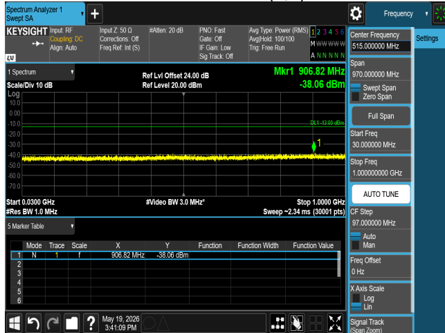
CSE n77 30M CH635666 BPSK(1,1)
