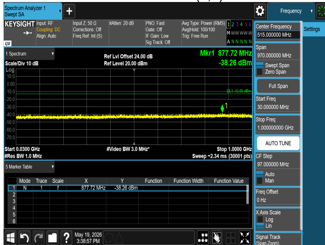
CSE n77 20M CH633334 BPSK(1,1)
