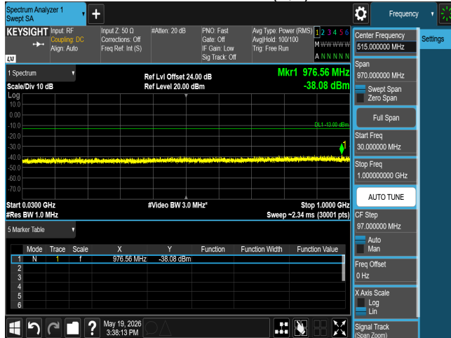
CSE n77 15M CH636166 BPSK(1,1)
