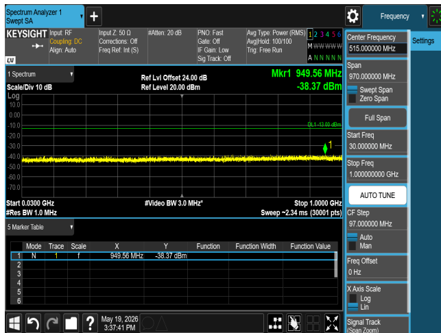
CSE n77 15M CH630500 BPSK(1,1)
