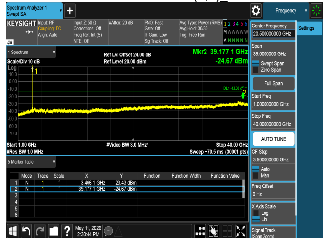
CSE n77 70M CH633334 BPSK(1,1)
