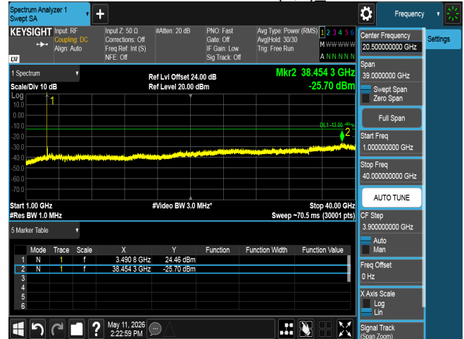
CSE n77 60M CH634666 BPSK(1,1)_
