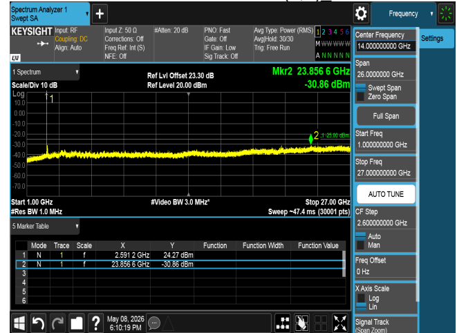
CSE n41 100M CH528000 BPSK(1,1)_
