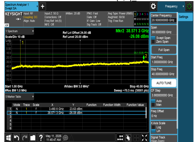
CSE n77 20M CH633334 BPSK(1,1)
