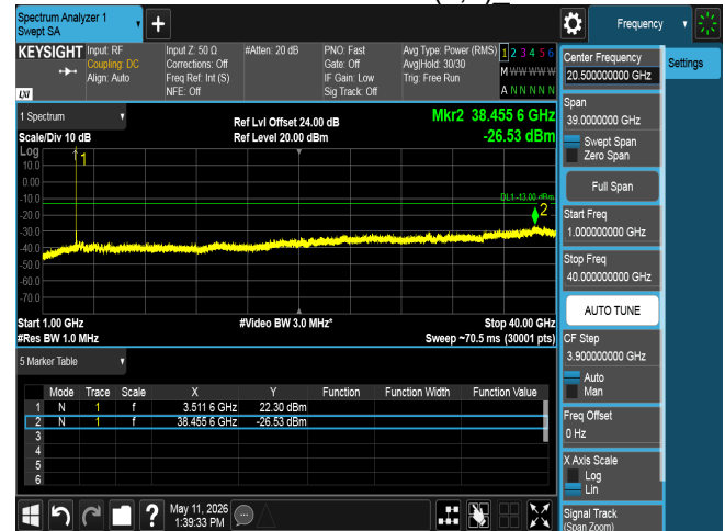
CSE n77 40M CH635332 BPSK(1,1)_
