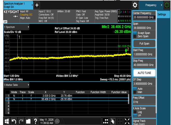
CSE n77 15M CH636166 BPSK(1,1)_
