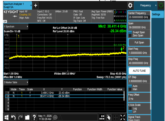
CSE n77 25M CH633334 BPSK(1,1)
