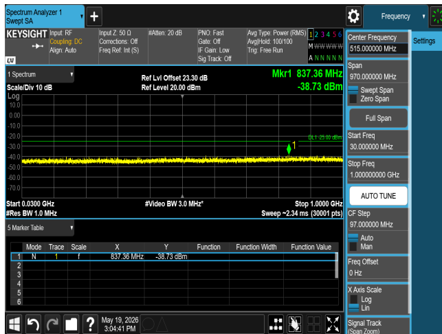
CSE n41 100M CH509202 BPSK(1,1)
