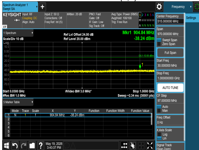
CSE n77 30M CH633334 BPSK(1,1)
