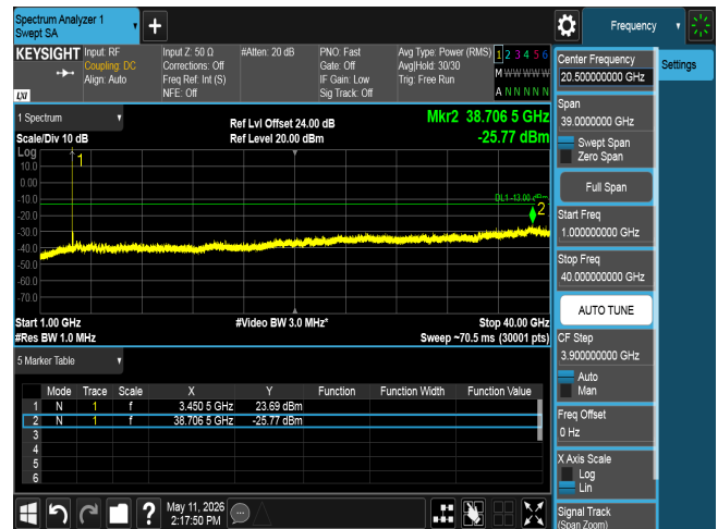
CSE n77 60M CH632000 BPSK(1,1)
