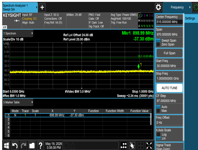
CSE n77 20M CH630668 BPSK(1,1)
