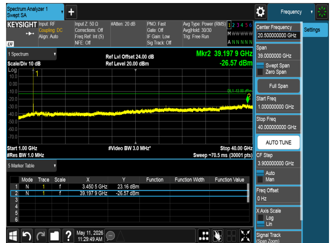
CSE n77 15M CH630500 BPSK(1,1)
