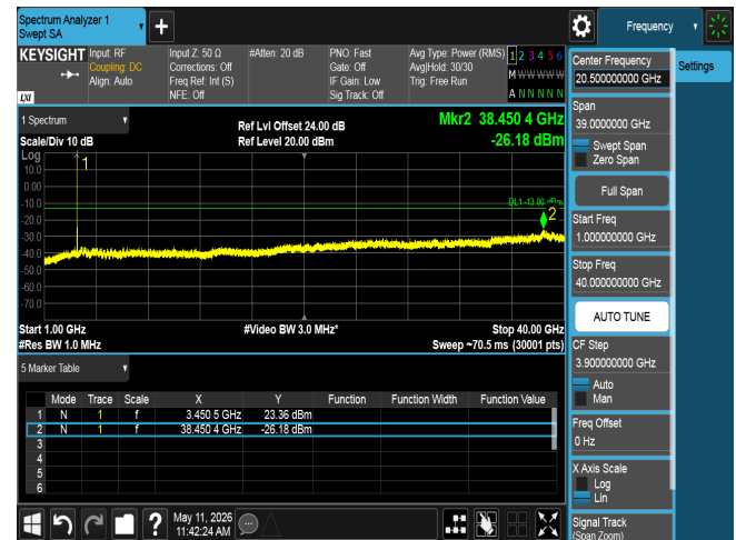
CSE n77 20M CH630668 BPSK(1,1)
