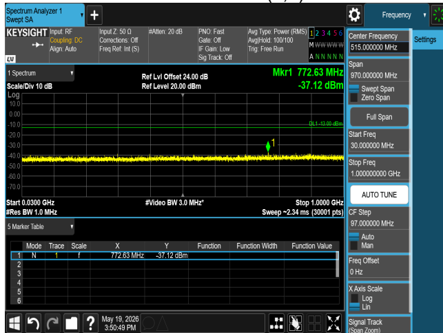
CSE n77 70M CH634332 BPSK(1,1)
