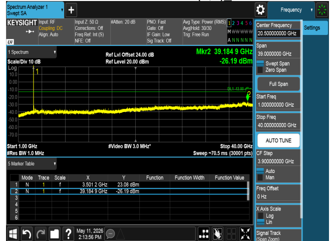
CSE n77 50M CH635000 BPSK(1,1)_
