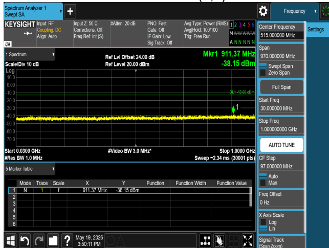
CSE n77 70M CH633334 BPSK(1,1)
