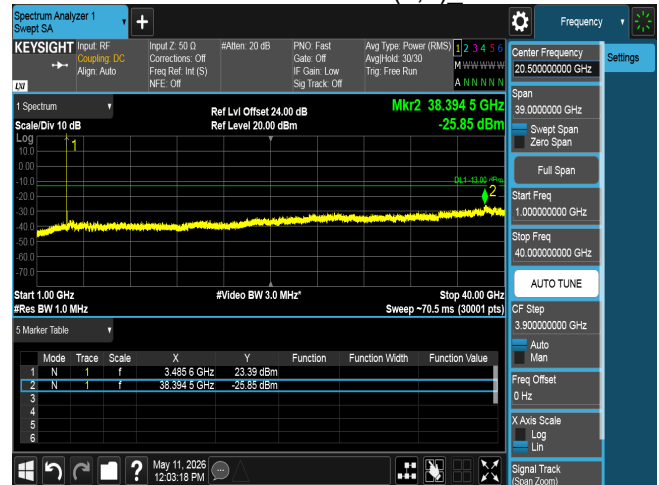
CSE n77 30M CH633334 BPSK(1,1)
