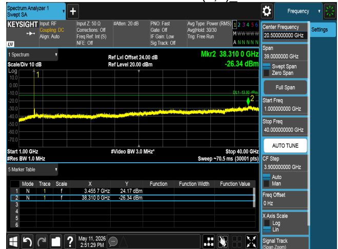
CSE n77 90M CH633334 BPSK(1,1)
