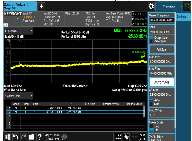
CSE n77 80M CH633334 BPSK(1,1)
