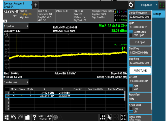
CSE n77 90M CH633666 BPSK(1,1)_
