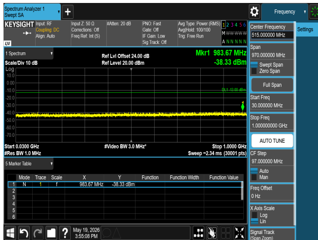
CSE n77 90M CH633000 BPSK(1,1)
