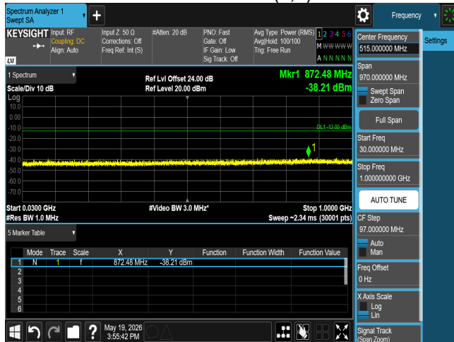
CSE n77 90M CH633334 BPSK(1,1)
