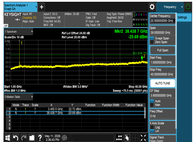
CSE n77 80M CH632668 BPSK(1,1)
