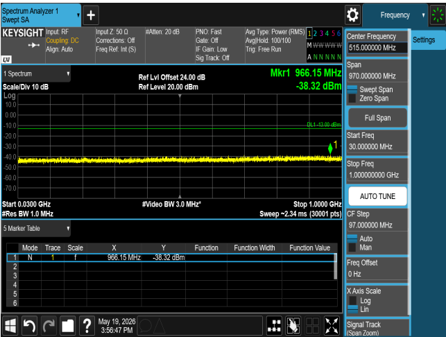
CSE n77 100M CH633334 BPSK(1,1)
