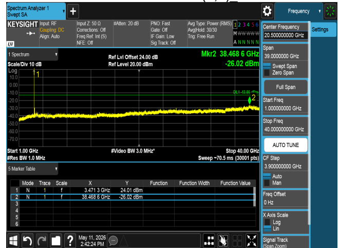
CSE n77 80M CH634000 BPSK(1,1)_
