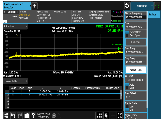
CSE n77 90M CH633000 BPSK(1,1)
