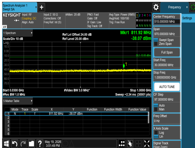
CSE n77 80M CH632668 BPSK(1,1)
