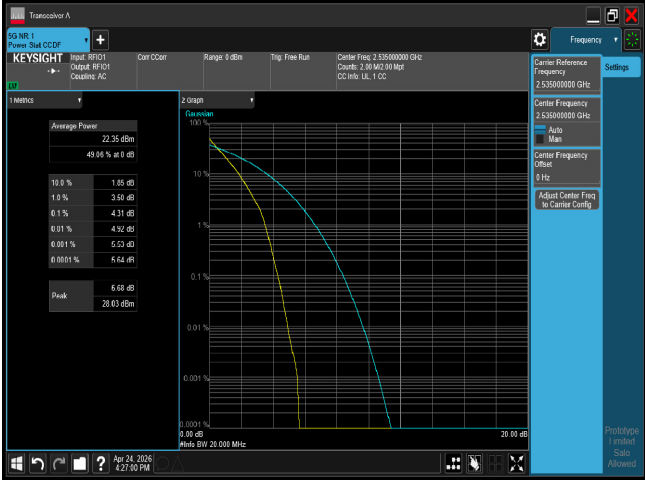
PTAR n7 20M CH507000 BPSK
