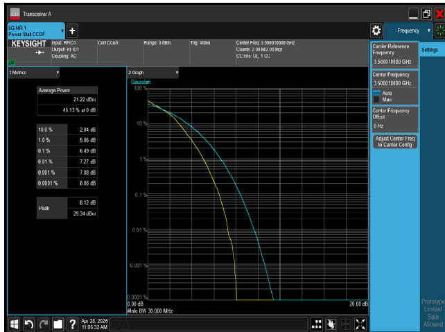
PTAR n77 30M CH633334 16QAM
