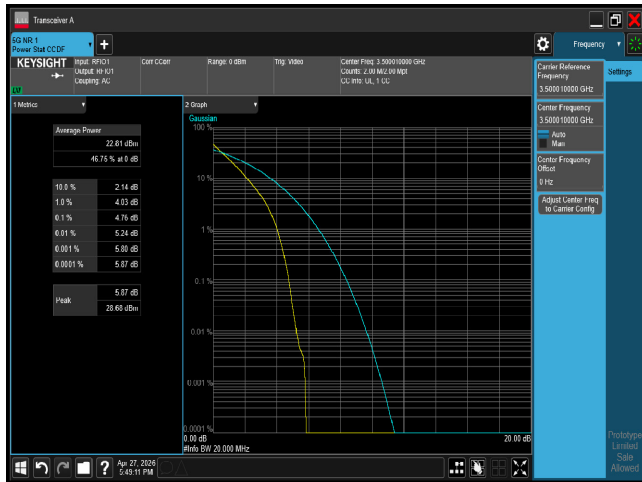
PTAR n77 20M CH633334 BPSK
