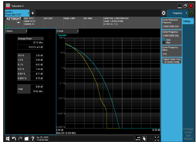
PTAR n77 30M CH633334 64QAM
