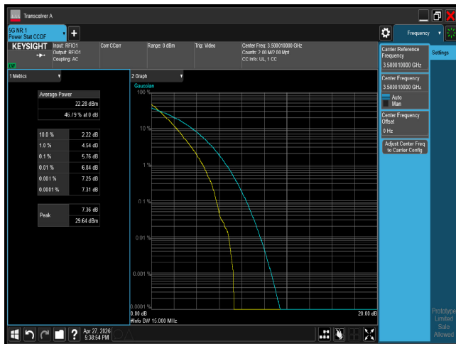
PTAR n77 15M CH633334 QPSK
