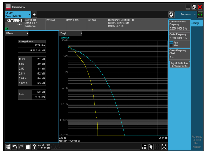
PTAR n77 40M CH633334 BPSK
