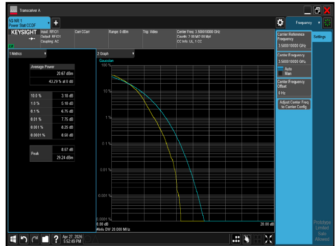
PTAR n77 20M CH633334 64QAM
