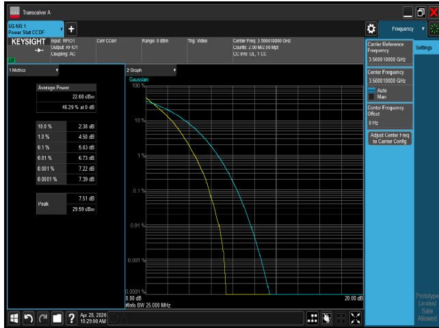
PTAR n77 25M CH633334 QPSK
