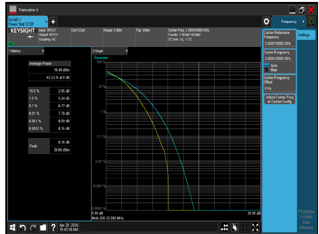
PTAR n77 25M CH633334 256QAM
