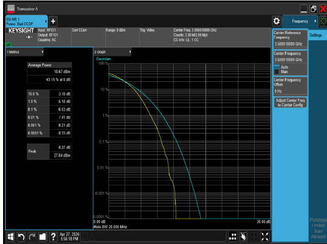
PTAR n77 20M CH633334 256QAM
