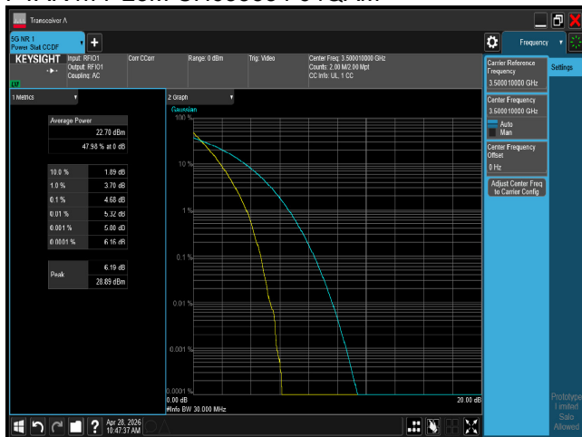
PTAR n77 30M CH633334 BPSK
