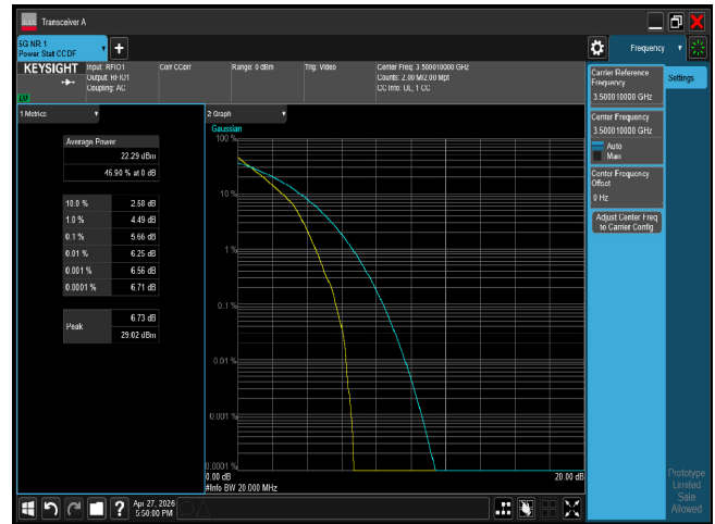
PTAR n77 20M CH633334 QPSK
