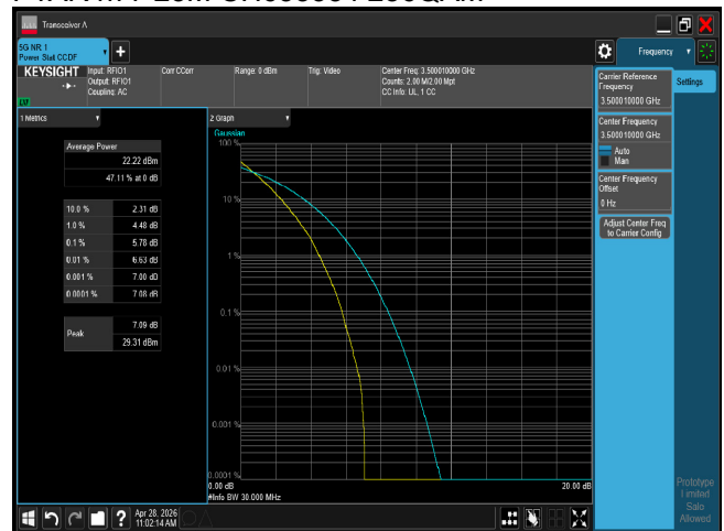
PTAR n77 30M CH633334 QPSK
