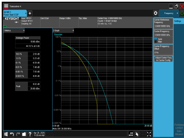
PTAR n77 30M CH633334 256QAM
