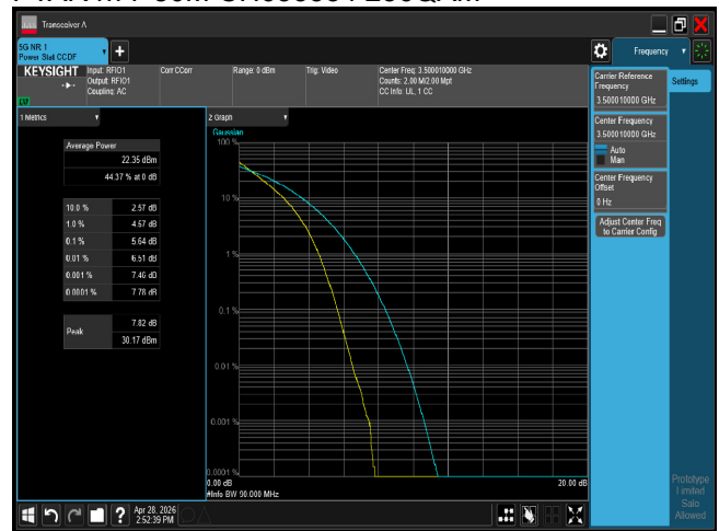
PTAR n77 90M CH633334 QPSK
