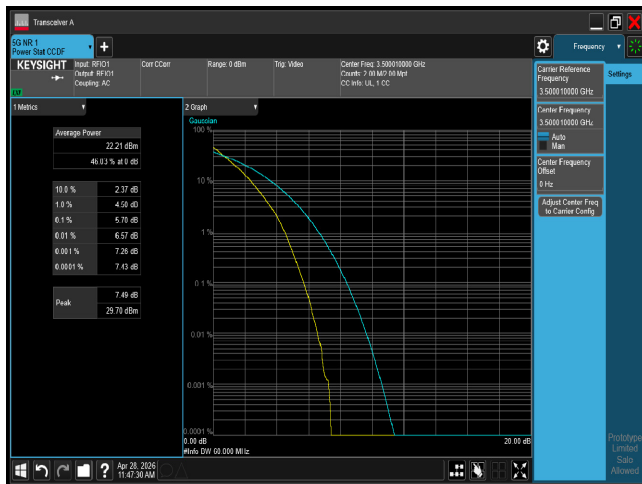
PTAR n77 60M CH633334 QPSK
