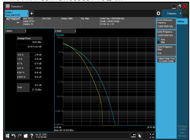
PTAR n77 60M CH633334 256QAM
