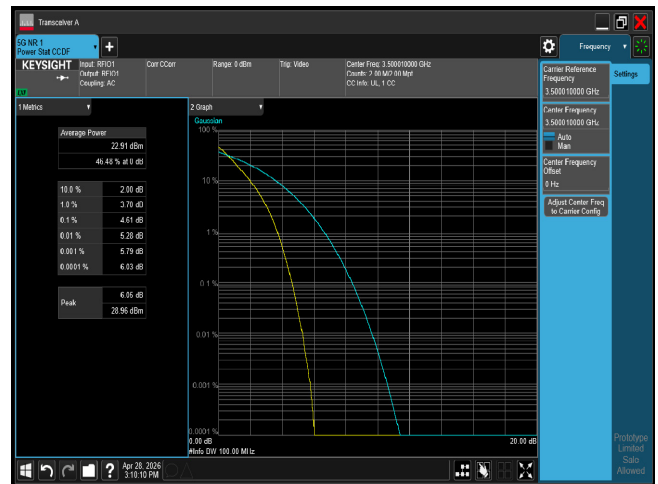
PTAR n77 100M CH633334 BPSK
