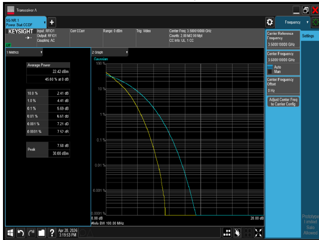
PTAR n77 100M CH633334 QPSK
