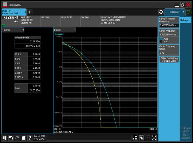
PTAR n77 70M CH633334 256QAM
