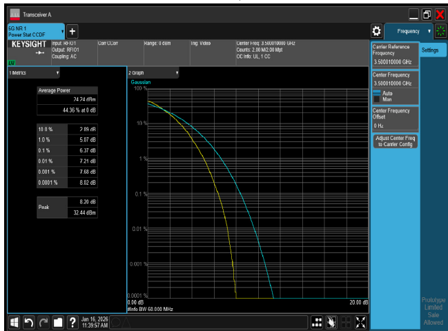
PTAR n77 60M CH633334 64QAM
