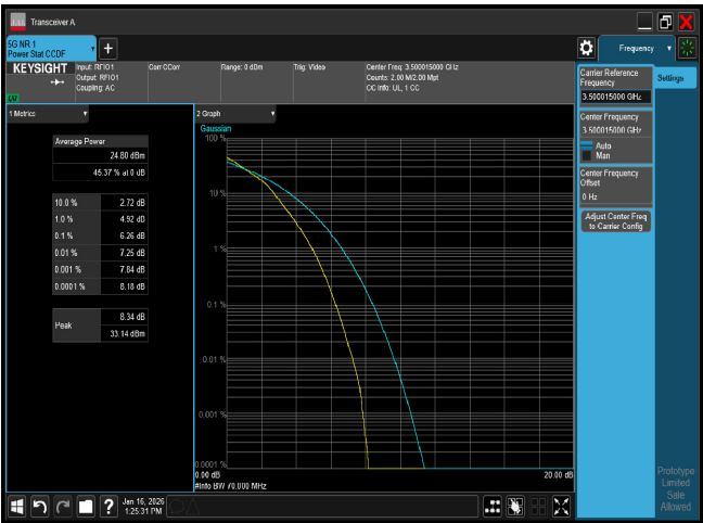
PTAR n77 70M CH633334 16QAM
