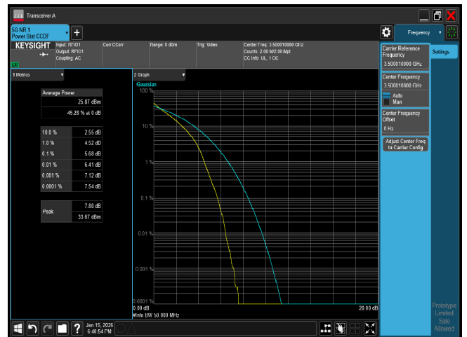
PTAR n77 50M CH633334 QPSK
