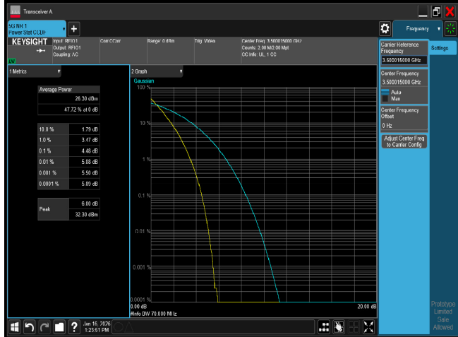
PTAR n77 70M CH633334 BPSK
