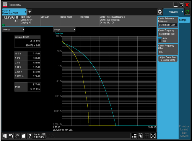
PTAR n77 80M CH633334 BPSK
