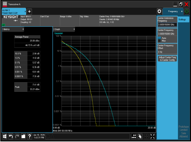
PTAR n77 80M CH633334 QPSK
