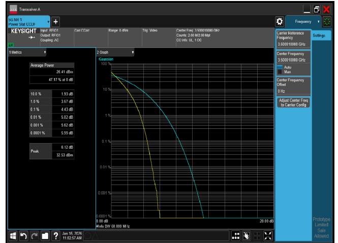
PTAR n77 60M CH633334 BPSK
