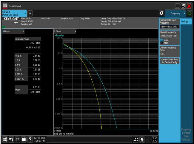
PTAR n77 70M CH633334 64QAM
