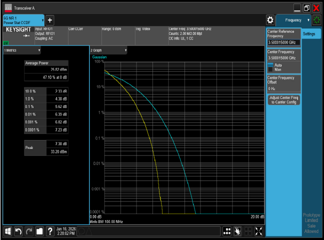
PTAR n77 100M CH633334 QPSK
