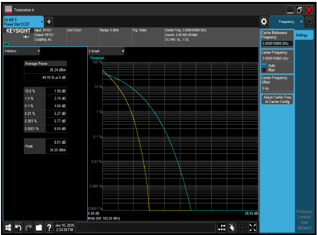
PTAR n77 100M CH633334 BPSK
