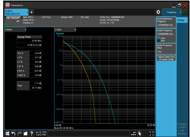
PTAR B77 20M CH656000 QPSK
