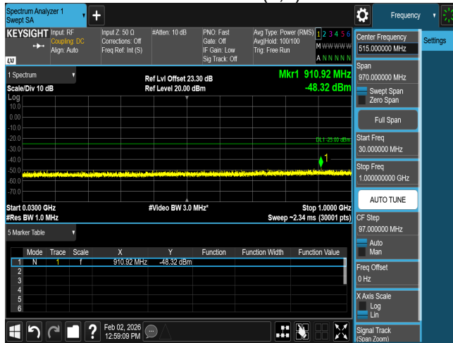
CSE n7 30M CH507000 BPSK(1,1)
