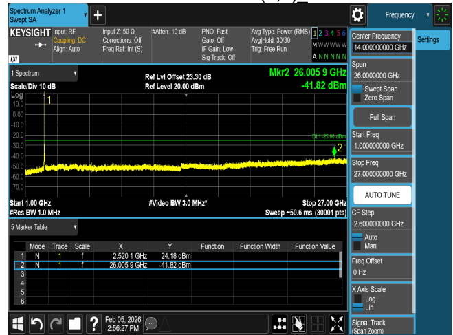
CSE n7 30M CH507000 BPSK(1,1)
