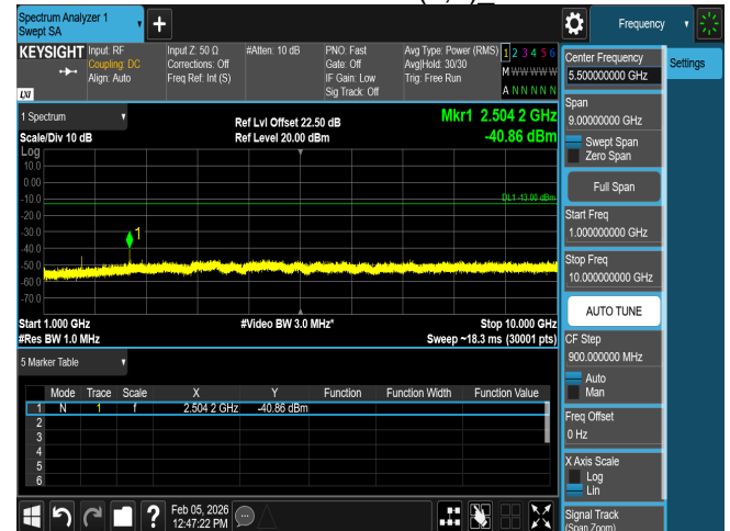
CSE n5 15M CH168300 BPSK(1,1)_
