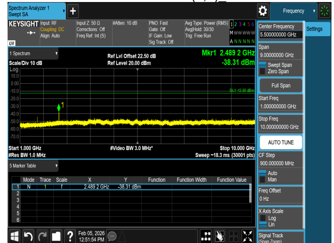
CSE n5 20M CH167800 BPSK(1,1)_
