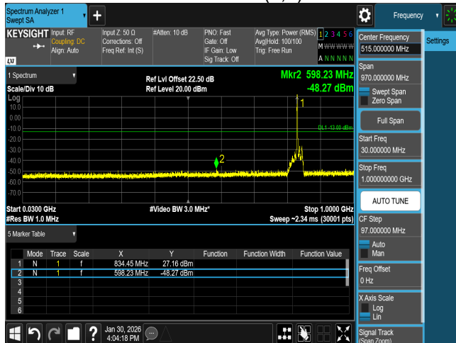
CSE n5 15M CH168300 BPSK(1,1)
