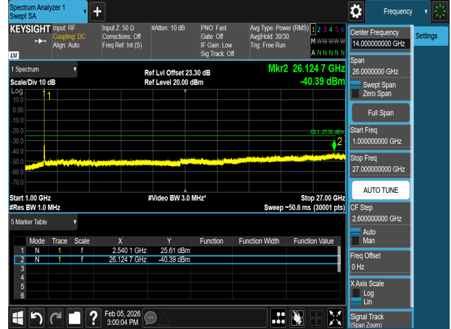
CSE n7 30M CH511000 BPSK(1,1)_
