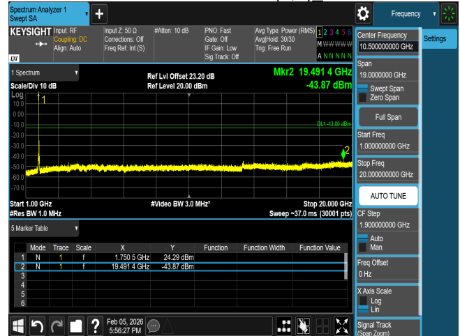
CSE n66 30M CH353000 BPSK(1,1)_
