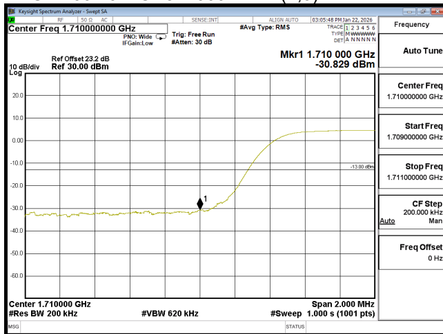
EDGE n66 20M CH344000 BPSK(100,0)
