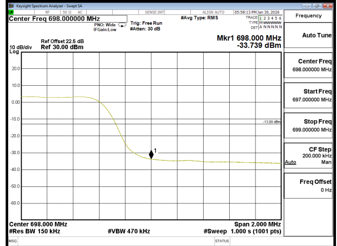
EDGE n71 15M CH138100 BPSK(75,4)
