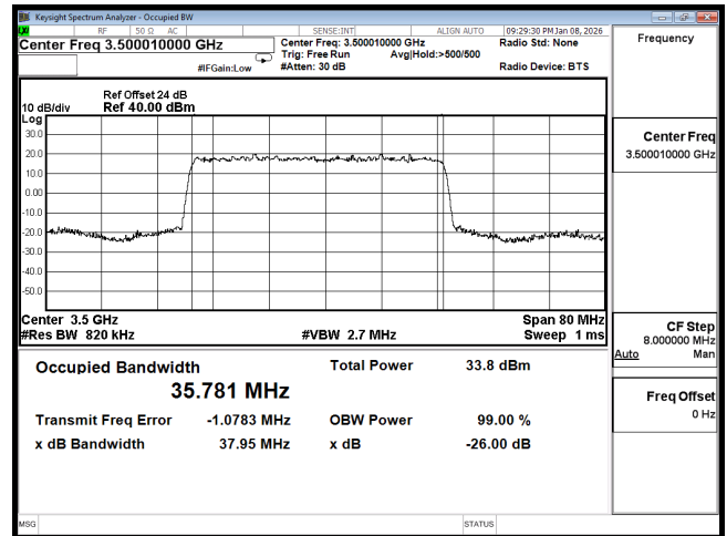
OCC n77 40M CH633334 BPSK
