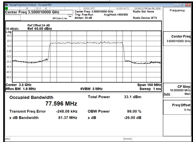
OCC n77 80M CH633334 BPSK
