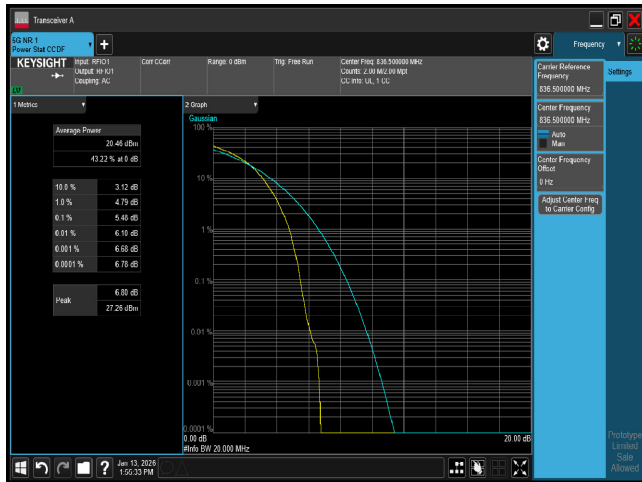
PTAR n5 20M CH167300 QPSK
