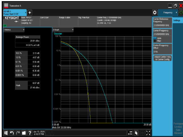
PTAR n7 20M CH507000 QPSK
