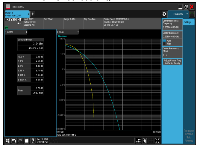
PTAR n7 20M CH507000 BPSK
