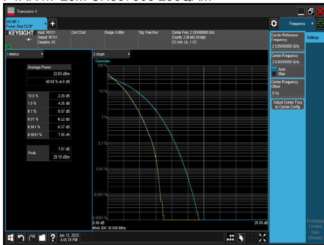
PTAR n7 30M CH507000 QPSK
