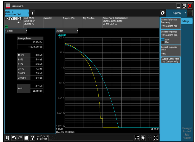
PTAR n7 20M CH507000 16QAM
