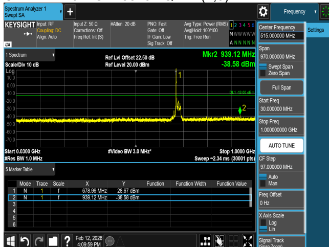
CSE B71 20M CH133372 QPSK(1,0)
