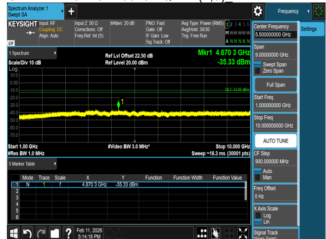
CSE B71 20M CH133372 QPSK(1,0)_
