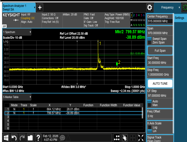
CSE B71 20M CH133222 QPSK(1,0)
