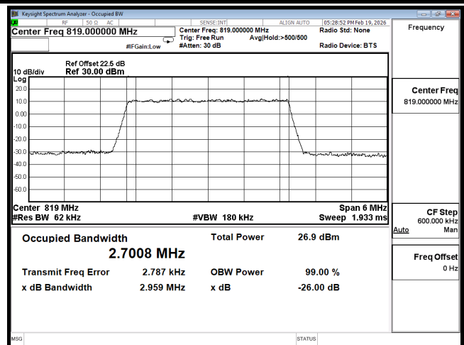
OCC B26 3M CH26740 256QAM
