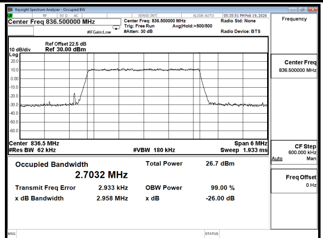
OCC B26 3M CH26915 256QAM
