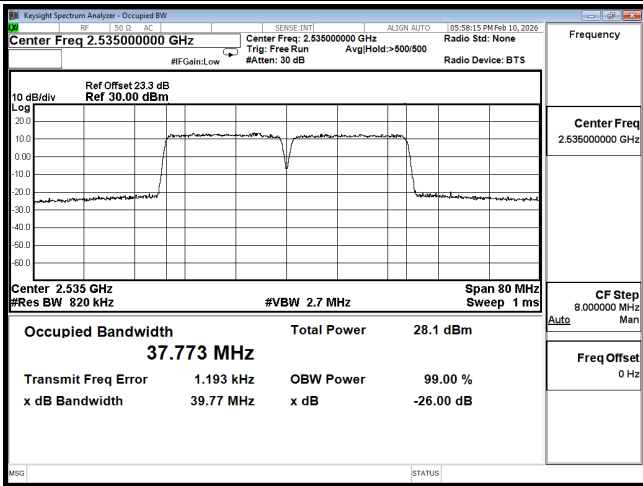
OOC B7 20M CH21001(100,0),20M CH21199(100,0) 16QAM
