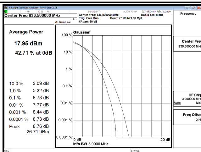
PTAR B26 3M CH26915 256QAM
