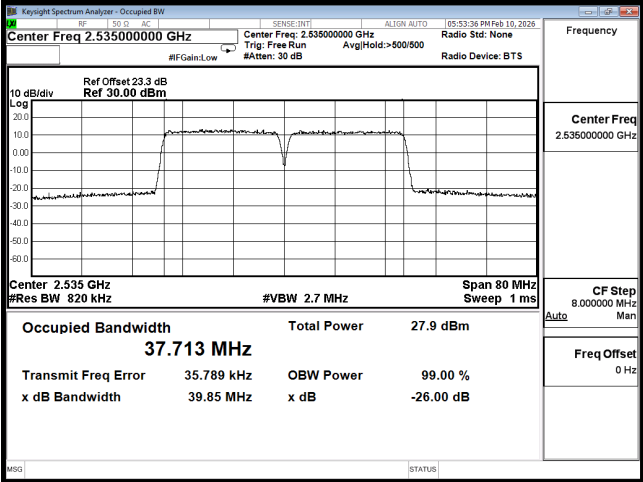
OOC B7 20M CH21001(100,0),20M CH21199(100,0) 64QAM
