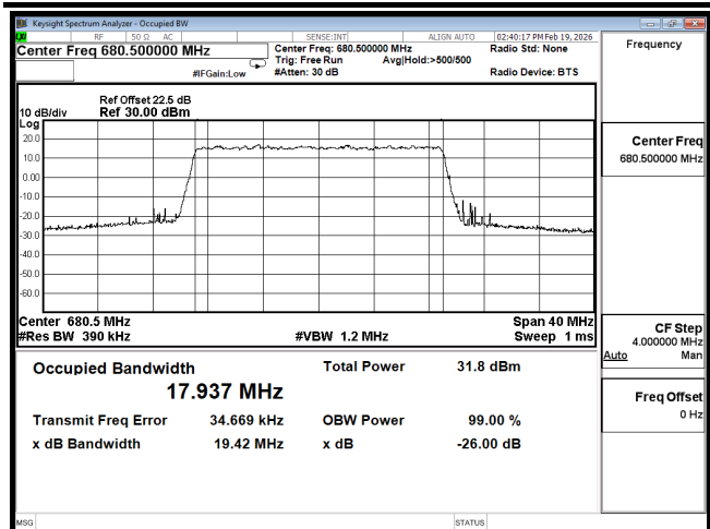
OCC B71 20M CH133297 QPSK
