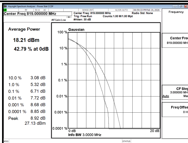
PTAR B26 3M CH26740 256QAM
