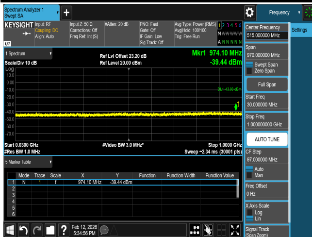
CSE B66 20M CH132072 QPSK(1,0)
