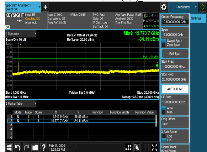
CSE B66 5M CH132322 QPSK(1,0)
