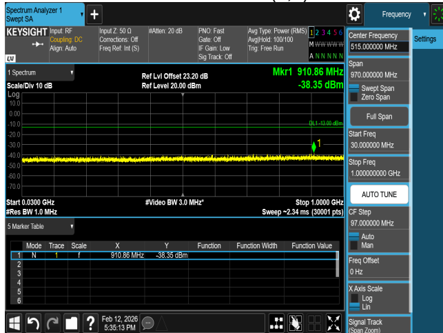
CSE B66 20M CH132322 QPSK(1,0)
