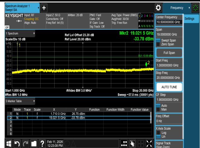
CSE B66 5M CH131997 QPSK(1,0)
