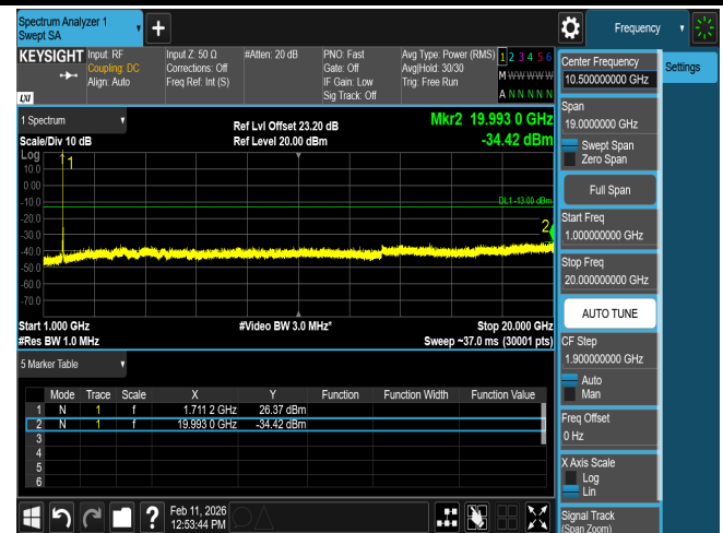
CSE B66 20M CH132072 QPSK(1,0)
