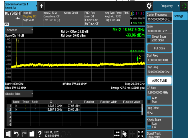
CSE B66 20M CH132322 QPSK(1,0)
