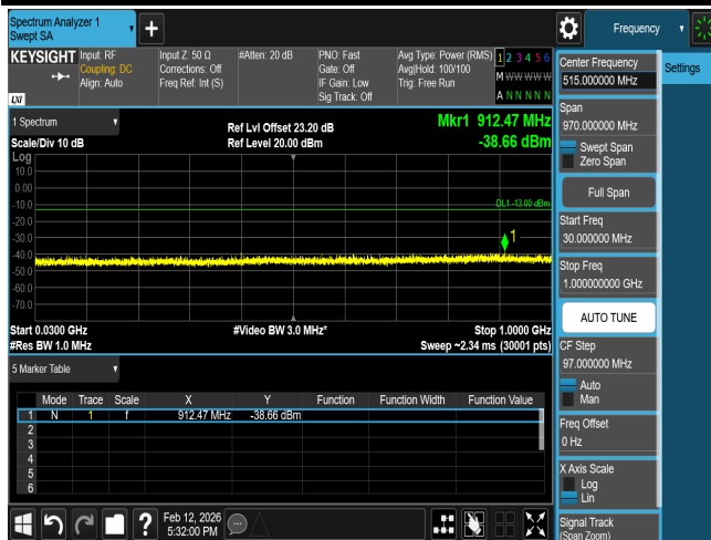
CSE B66 5M CH131997 QPSK(1,0)
