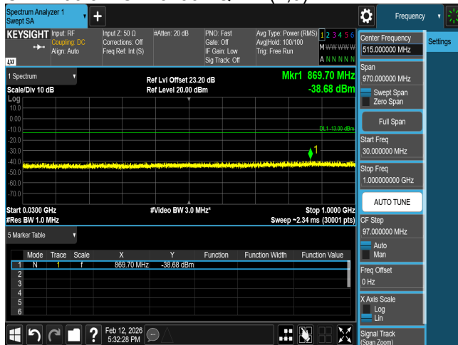
CSE B66 5M CH132322 QPSK(1,0)
