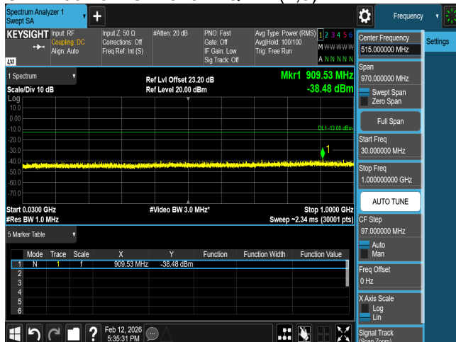
CSE B66 20M CH132572 QPSK(1,0)
