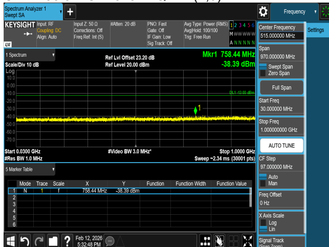
CSE B66 5M CH132647 QPSK(1,0)
