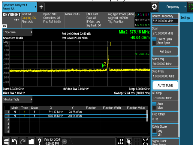
CSE B12 5M CH23095 QPSK(1,0)
