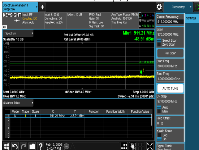
CSE B7 20M CH21350 QPSK(1,0)
