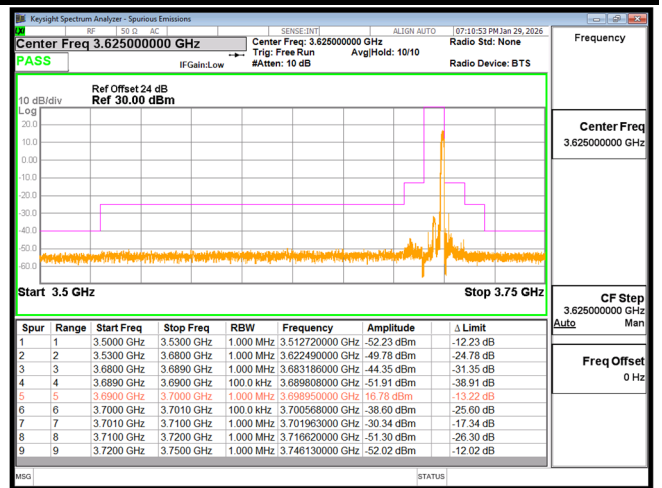
EDGE n48 10M CH646332 BPSK(1,23)
