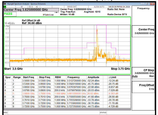
EDGE B48 20M CH56640 QPSK(1,0)
