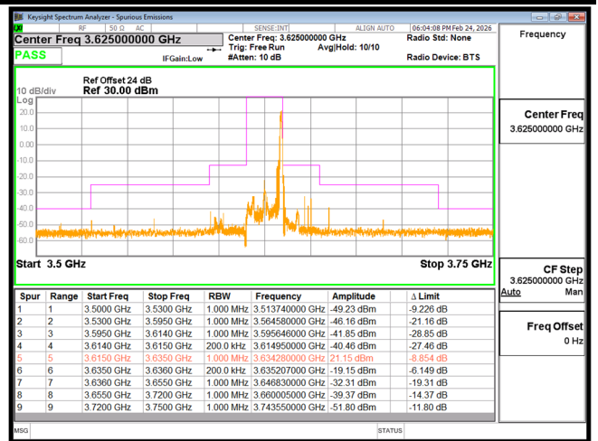
EDGE B48 20M CH55990 QPSK(1,99)
