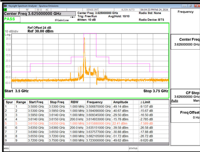
EDGE B48 20M CH55990 QPSK(1,0)
