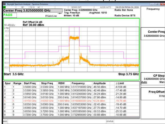
EDGE B48 20M CH55990 QPSK(100,0)
