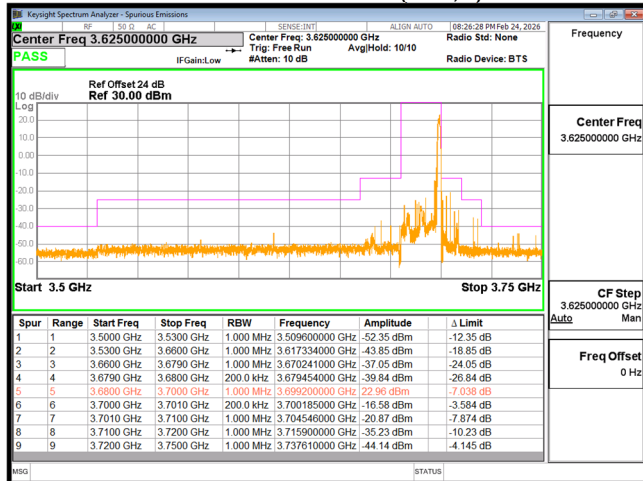
EDGE B48 20M CH56640 QPSK(1,99)
