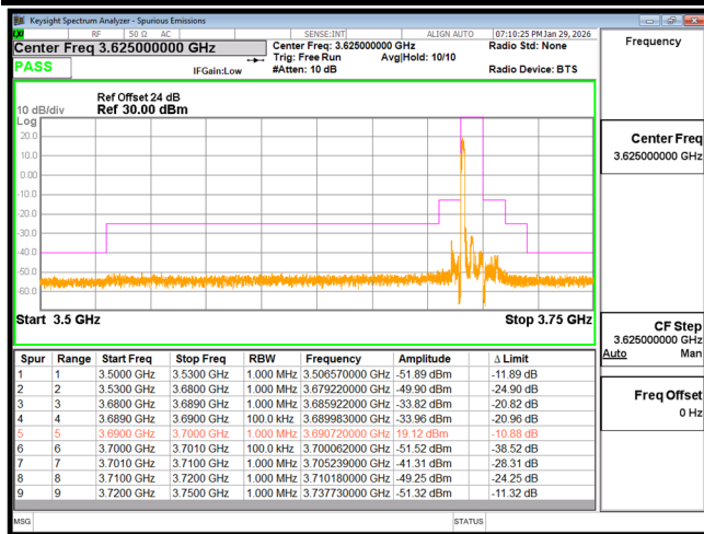
EDGE n48 10M CH646332 BPSK(1,0)
