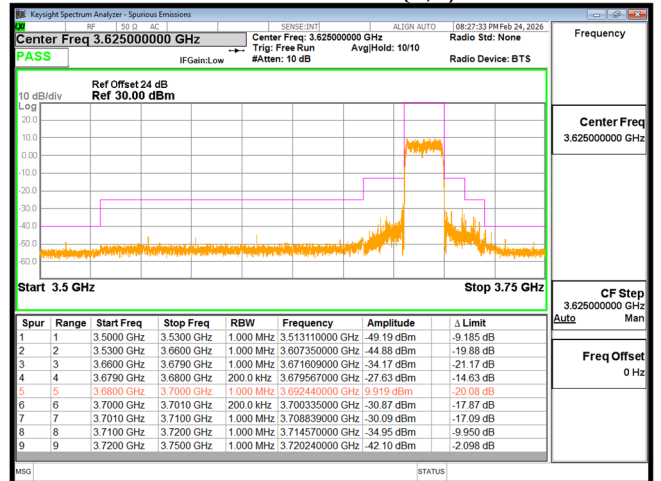
EDGE B48 20M CH56640 QPSK(100,0)
