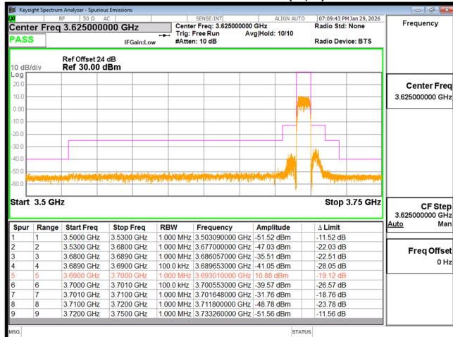
EDGE n48 10M CH646332 BPSK(24,0)
