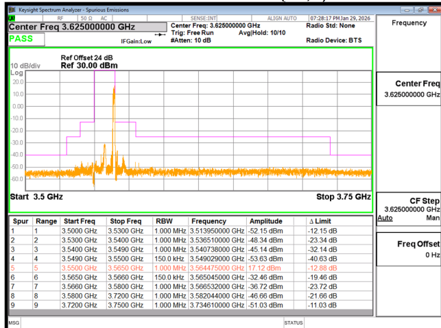
EDGE n48 15M CH637168 BPSK(1,37)
