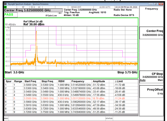
EDGE n48 40M CH638000 BPSK(1,0)
