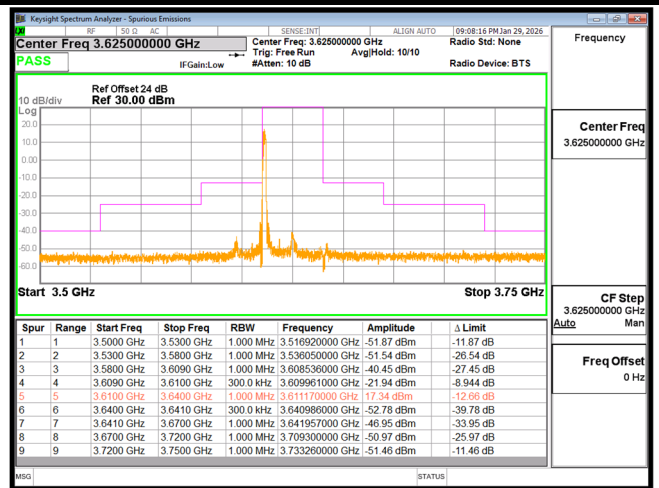
EDGE n48 30M CH641666 BPSK(1,0)
