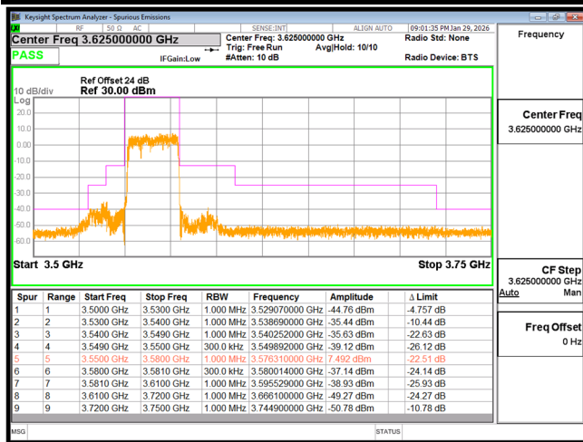
EDGE n48 30M CH637668 BPSK(75,3)
