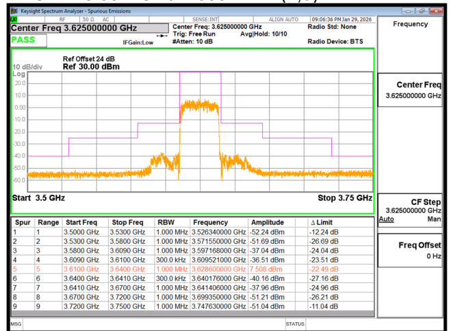
EDGE n48 30M CH641666 BPSK(75,0)
