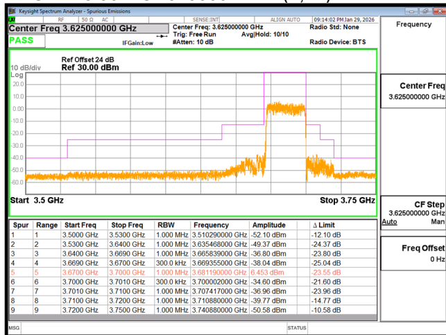
EDGE n48 30M CH645666 BPSK(75,3)
