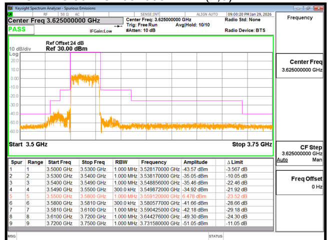
EDGE n48 30M CH637668 BPSK(75,0)
