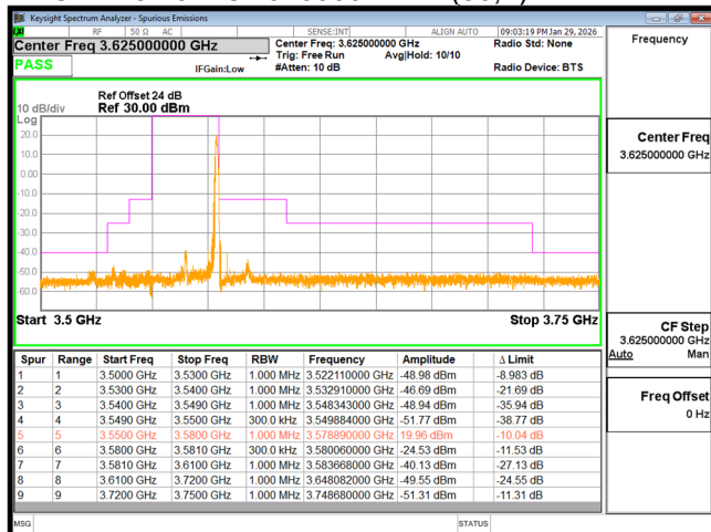
EDGE n48 30M CH637668 BPSK(1,77)
