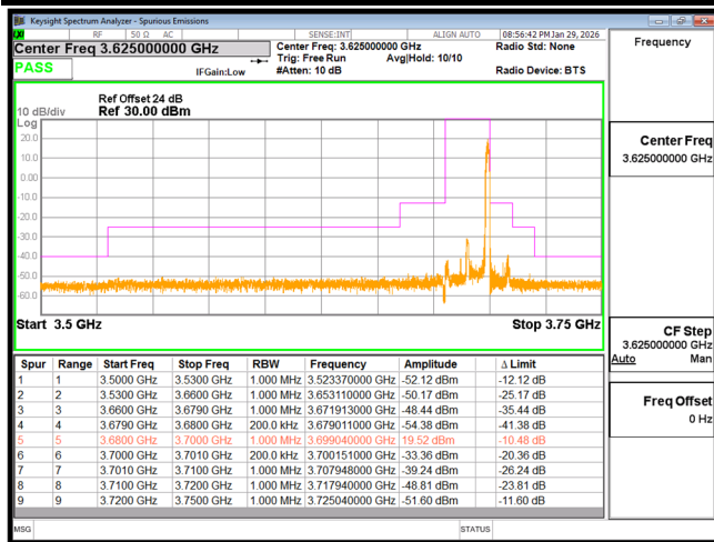
EDGE n48 20M CH646000 BPSK(1,50)
