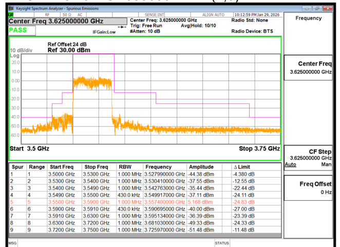
EDGE n48 40M CH638000 BPSK(100,0)
