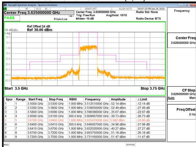
EDGE n48 30M CH641666 BPSK(75,3)
