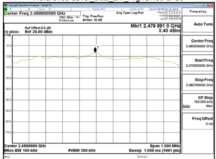
Reference Level BLE 2M HighCH39-2480
