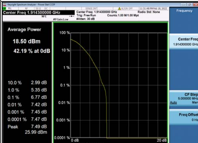
5MHz / 256QAM
