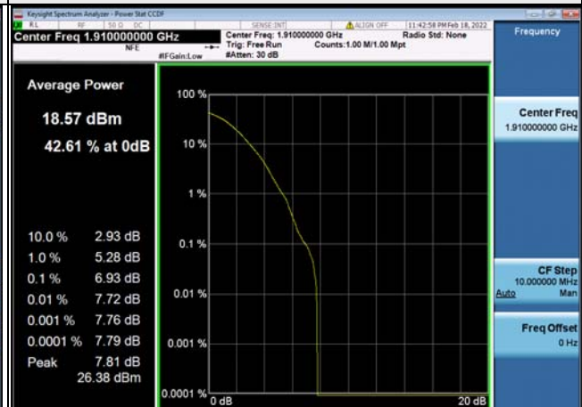
20MHz / 256QAM
