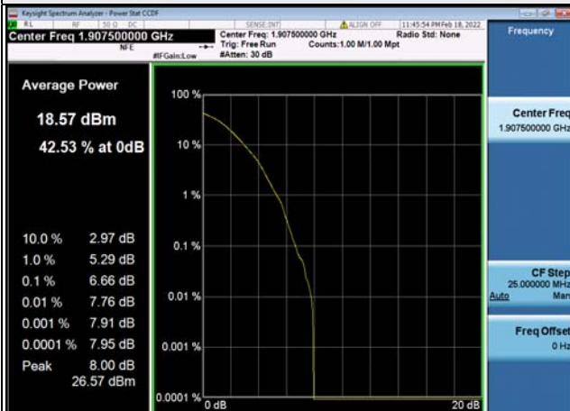
15MHz / 256QAM
