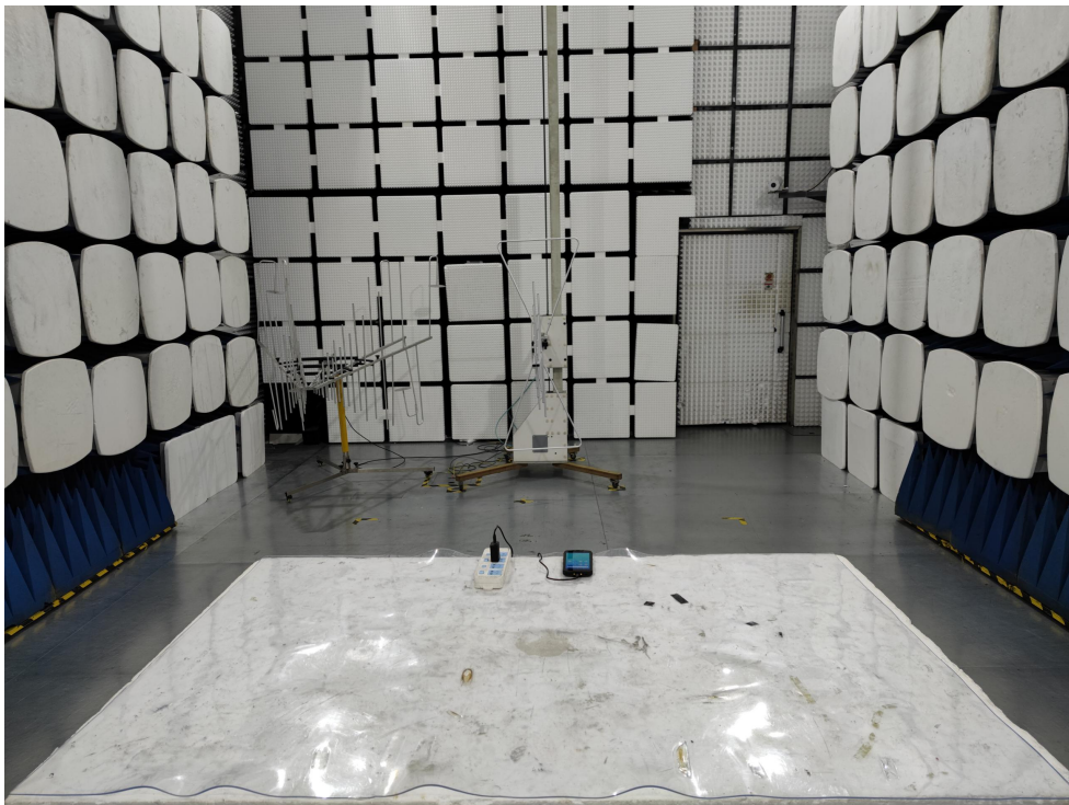
Fig. 2 (30MHz~1GHz)
