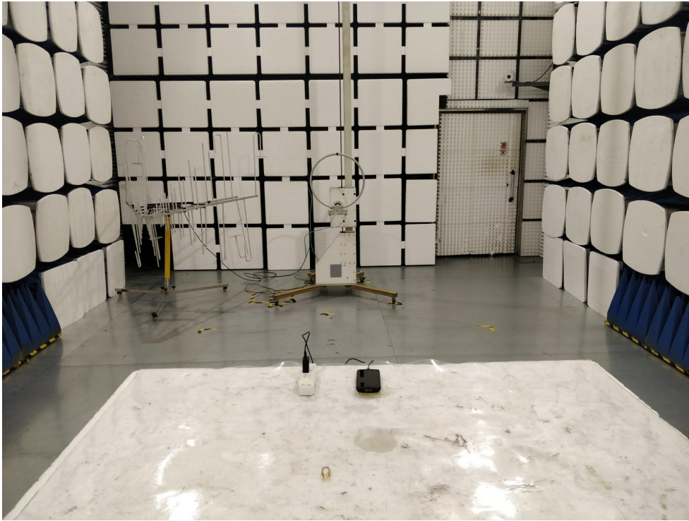
Fig. 1 (Below 30MHz)
