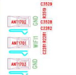
匹配电路
