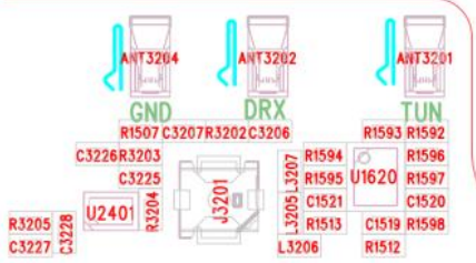
位号图
