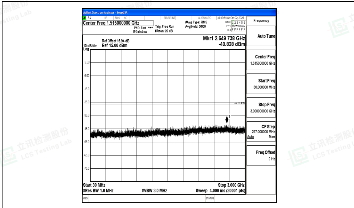
11AX80SISO-Ant0-5985-30~3000-PASS
