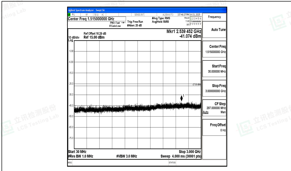
11AX80SISO-Ant0-6465-30~3000-PASS
