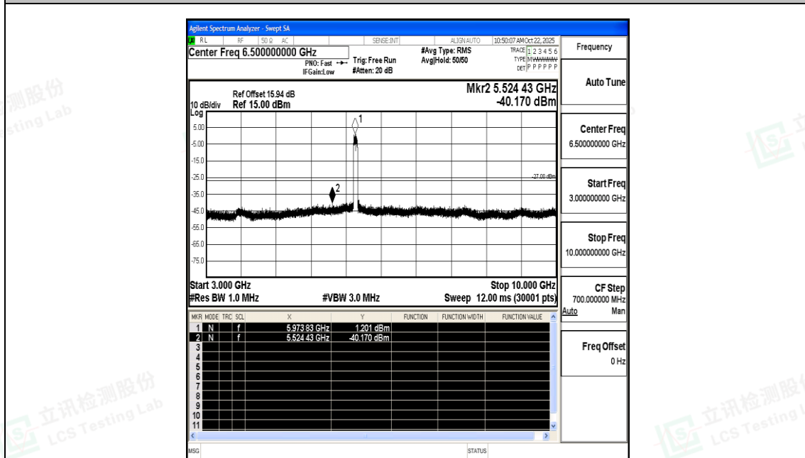
11AX80SISO-Ant0-5985-3000~10000-PASS
