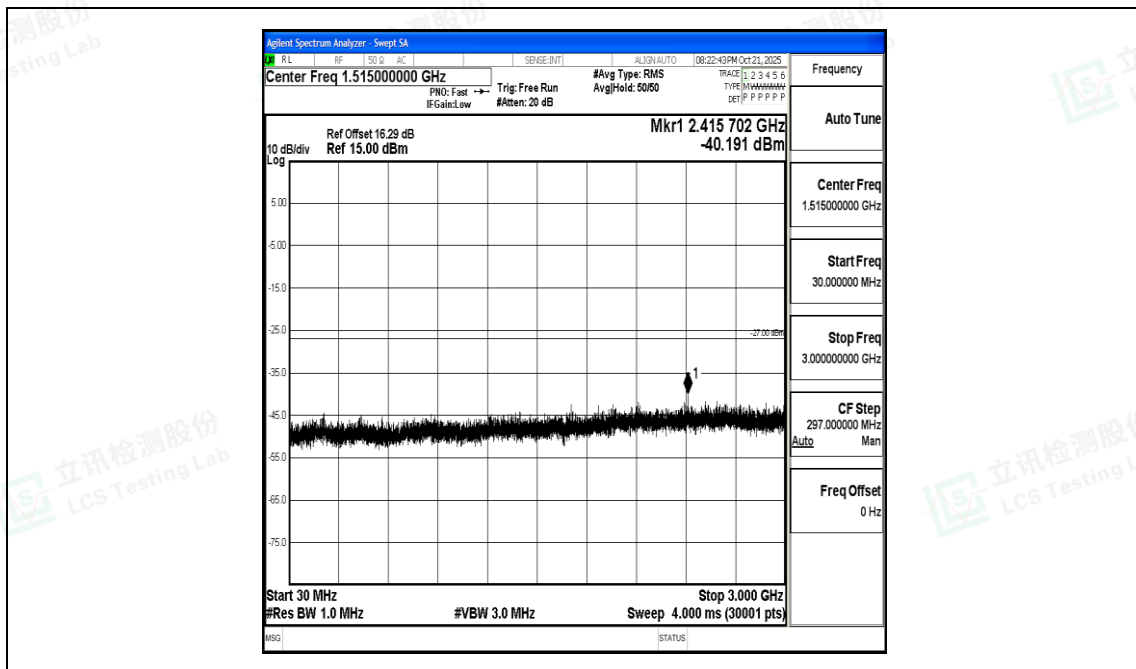
11AX80SISO-Ant1-6465-30~3000-PASS
