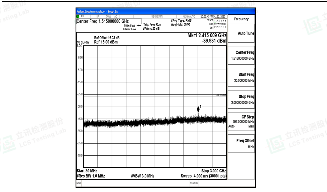
11AX80SISO-Ant0-6385-30~3000-PASS
