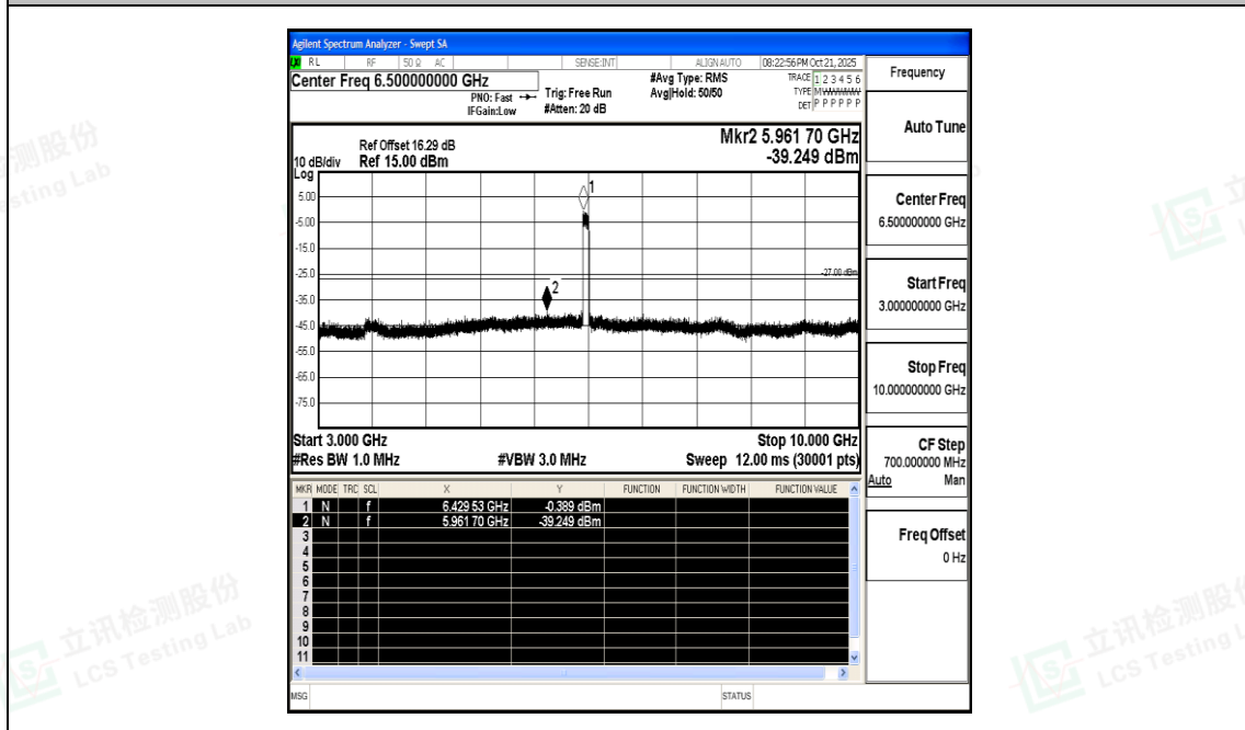
11AX80SISO-Ant1-6465-3000~10000-PASS
