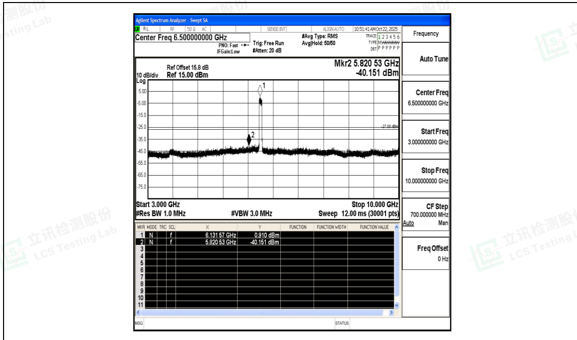
11AX80SISO-Ant0-6145-3000~10000-PASS
