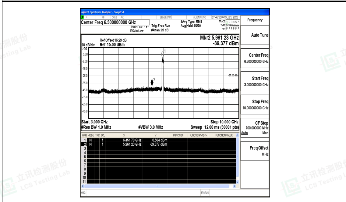
11AX80SISO-Ant0-6465-3000~10000-PASS
