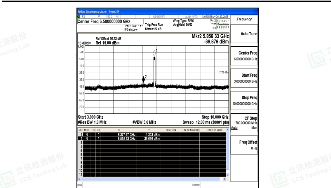
11AX80SISO-Ant0-6385-3000~10000-PASS
