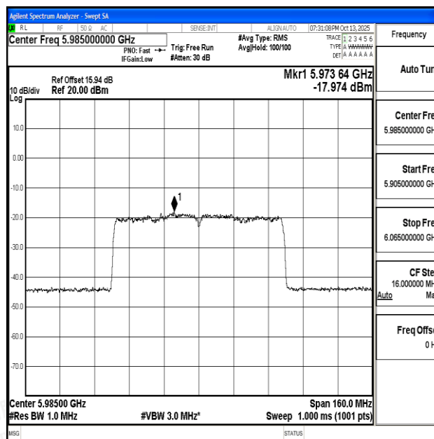
11AX80SISO-Ant1-5985-PASS
