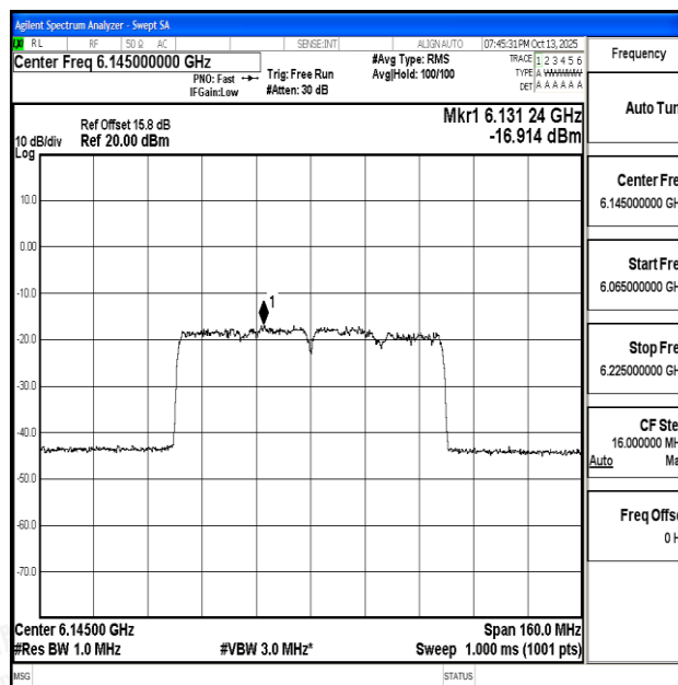
11AX80SISO-Ant0-6145-PASS
