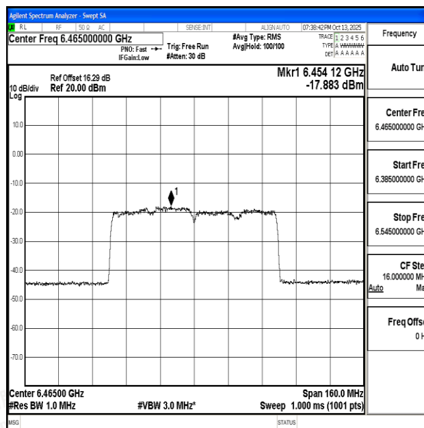
11AX80SISO-Ant1-6465-PASS
