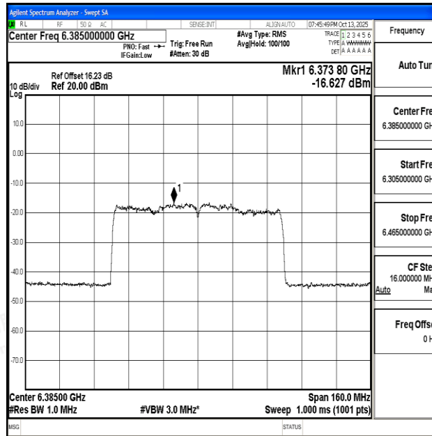
11AX80SISO-Ant0-6385-PASS
