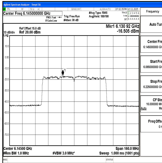
11AX80SISO-Ant1-6145-PASS
