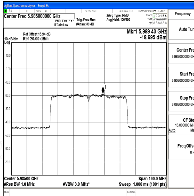
11AX80SISO-Ant0-5985-PASS
