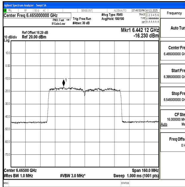
11AX80SISO-Ant0-6465-PASS
