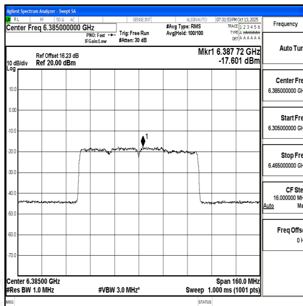
11AX80SISO-Ant1-6385-PASS
