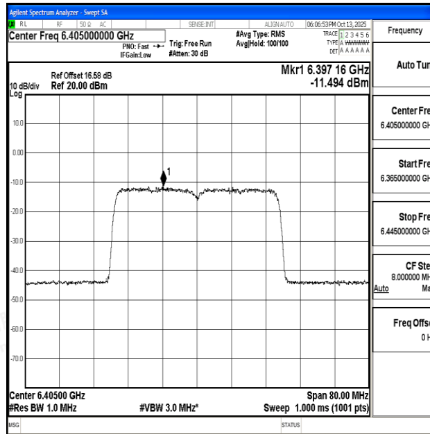
11AX40SISO-Ant1-6405-PASS
