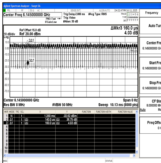
NTNV-11AX80SISO-Ant0-6145
