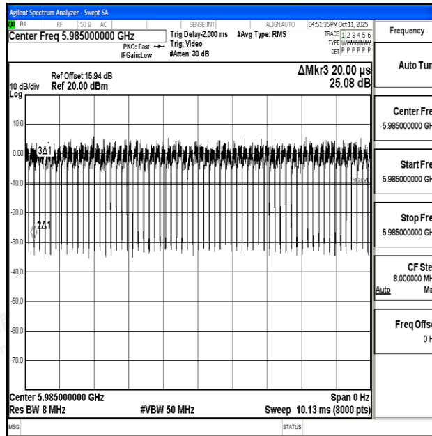
NTNV-11AX80SISO-Ant1-5985
