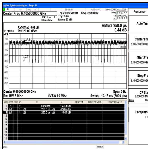
NTNV-11AX40SISO-Ant1-6405
