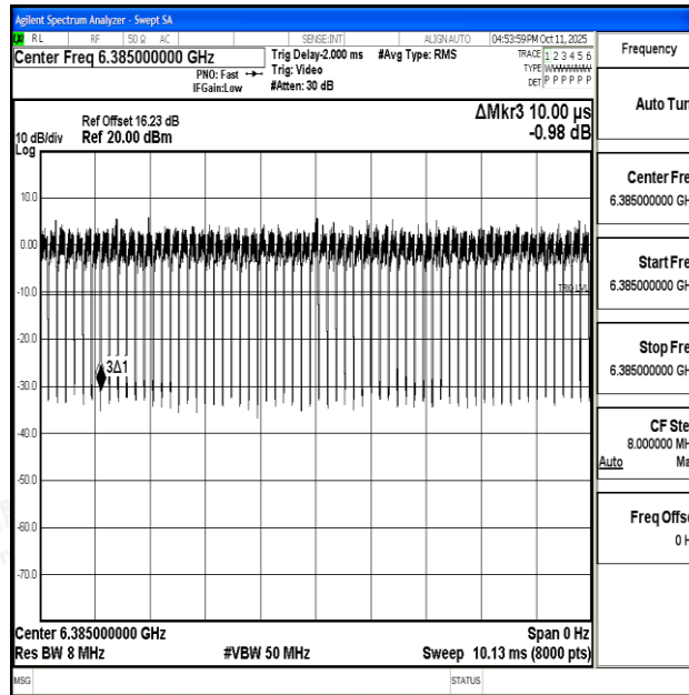
NTNV-11AX80SISO-Ant1-6385
