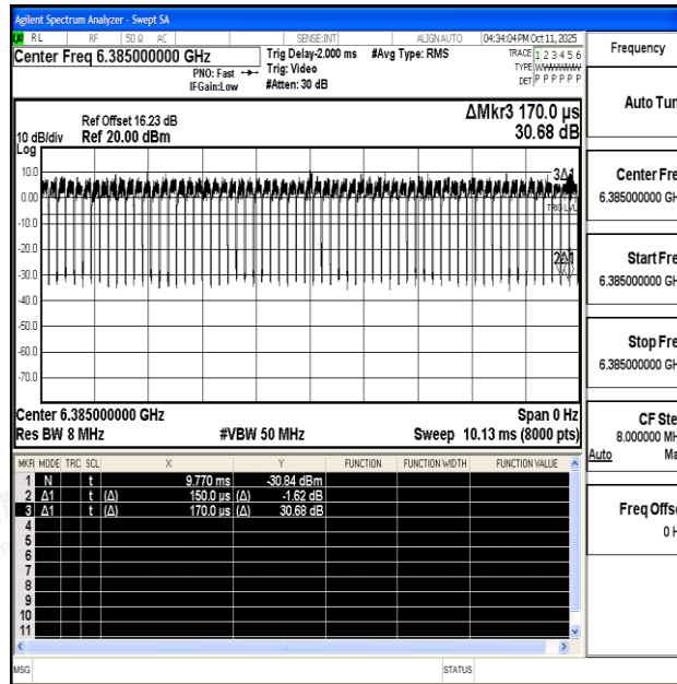
NTNV-11AX80SISO-Ant0-6385
