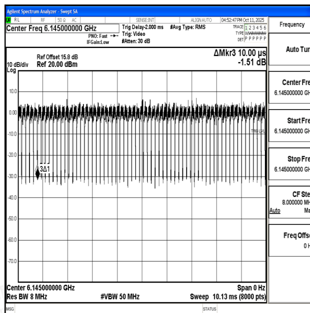
NTNV-11AX80SISO-Ant1-6145
