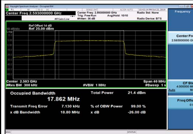
TDD41_MidRange_20MHz_2593MHz_QPSK
