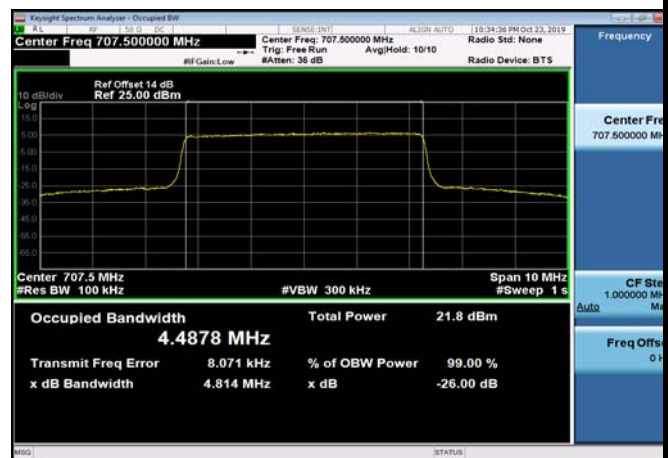
FDD12_MidRange_5MHz_707.5MHz_Q16
