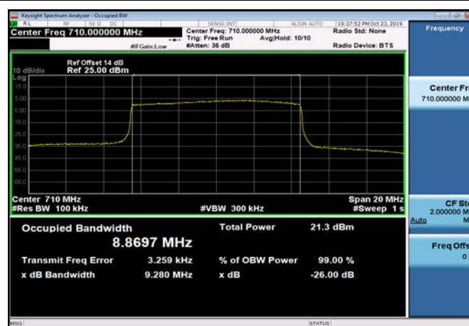
FDD17_MidRange_10MHz_710MHz_Q16
