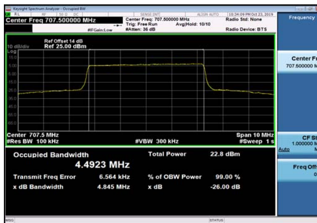
FDD12_MidRange_5MHz_707.5MHz_QPSK
