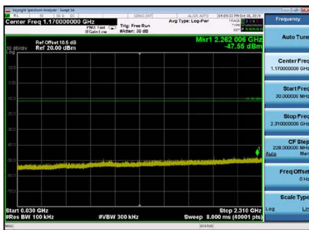
,Plot 3,30MHz~2310MHz-802.11b,2462MHz
