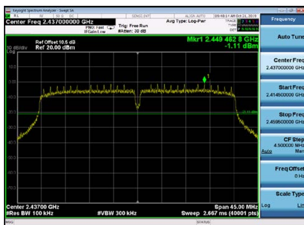
,Plot 1,Reference Level-802.11n(HT40) ,2437MHz
