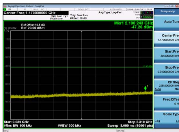
,Plot 3,30MHz~2310MHz-802.11n(HT40) ,2452MHz
