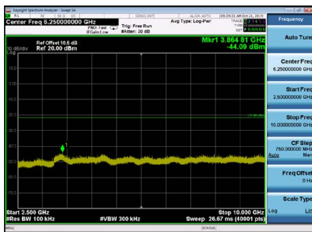
,Plot 4,2500MHz~10000MHz-802.11n(HT40 ) ,2452MHz
