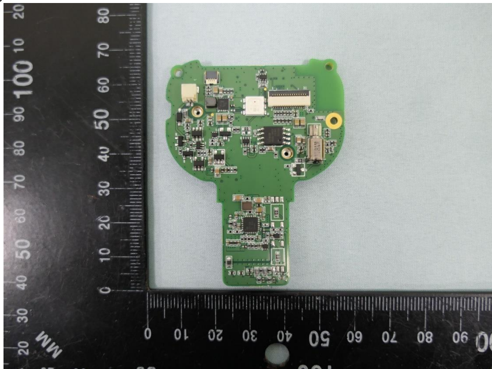
(18) EUT Photo
