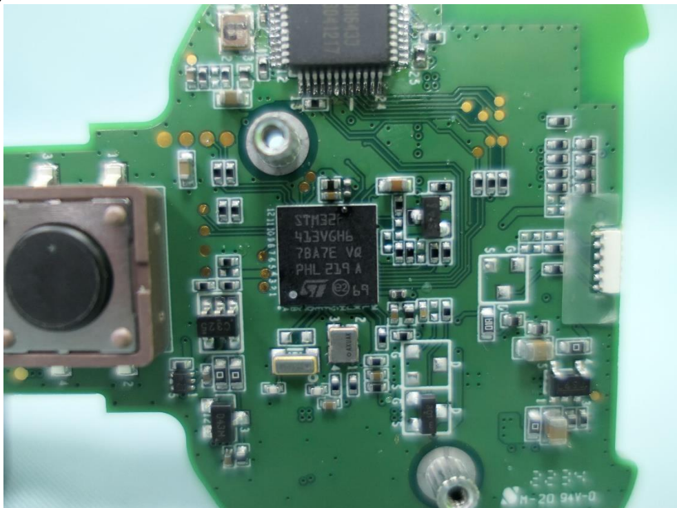
(16) EUT Photo
