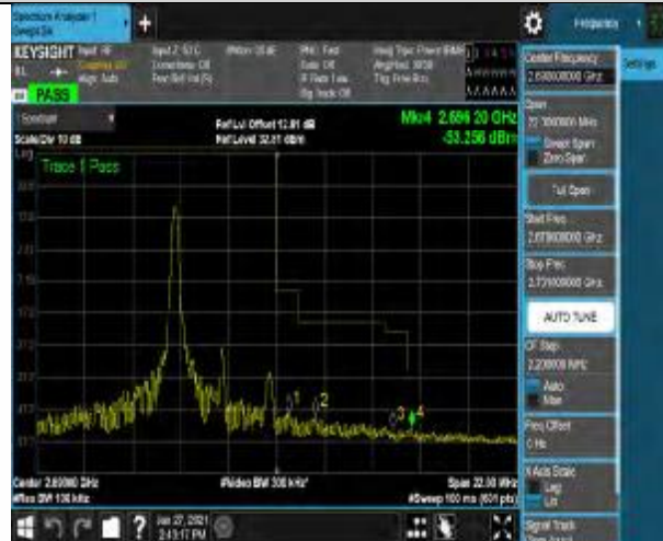
Band41-5MHz-16QAM-41565-1RB#24
