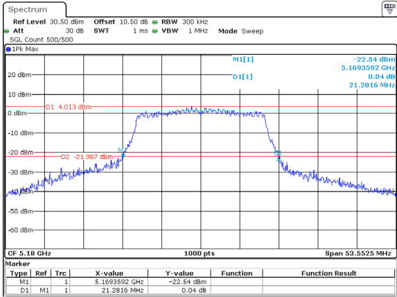
802.11ac20_5180MHz_ANT2
