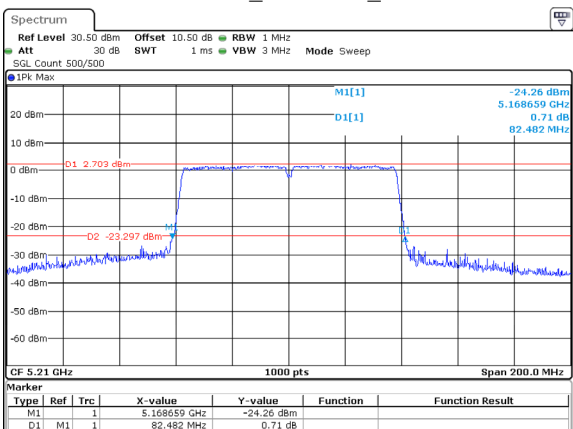
802.11ac80_5210MHz_ANT1
