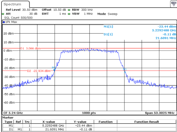
802.11ac20_5240MHz_ANT2
