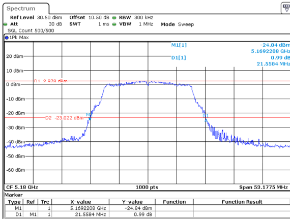
802.11a_5180MHz_ANT1
