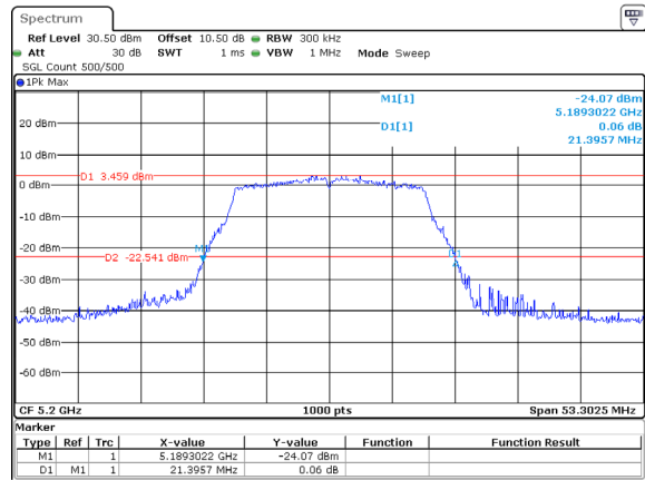
802.11a_5200MHz_ANT1
