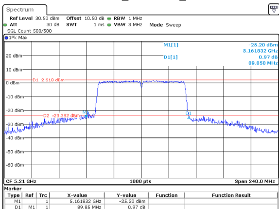
802.11ac80_5210MHz_ANT2
