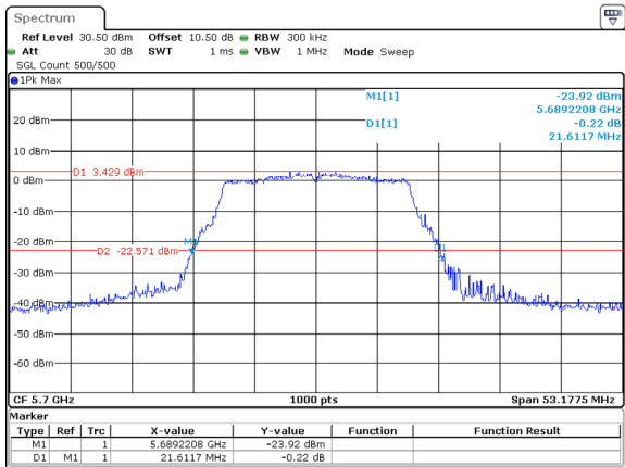
802.11a_5700MHz_ANT1
