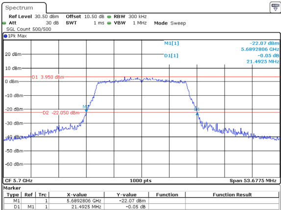
802.11ac20_5700MHz_ANT1
