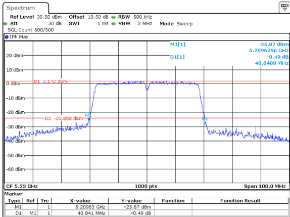
802.11ac40_5230MHz_ANT1
