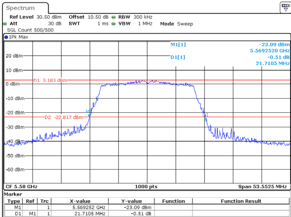
802.11ac20_5580MHz_ANT1
