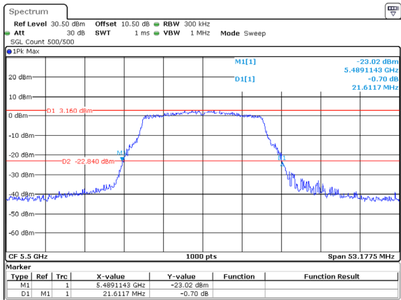
802.11a_5500MHz_ANT1
