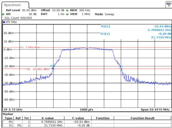
802.11a_5720MHz_ANT1
