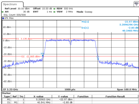
802.11ac40_5230MHz_ANT2
