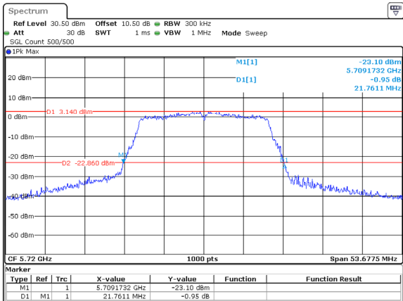
802.11ac20_5720MHz_ANT1
