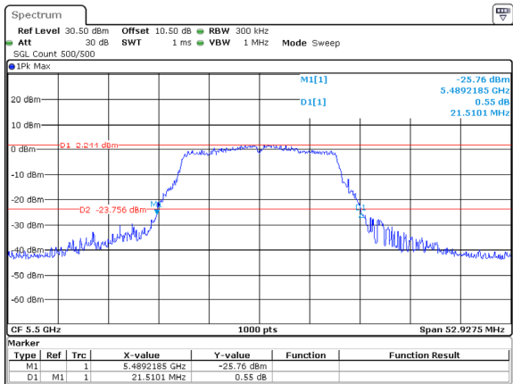
802.11a_5500MHz_ANT2
