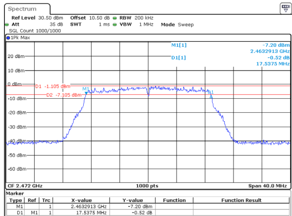
802.11n20_2472MHz_ANT1
