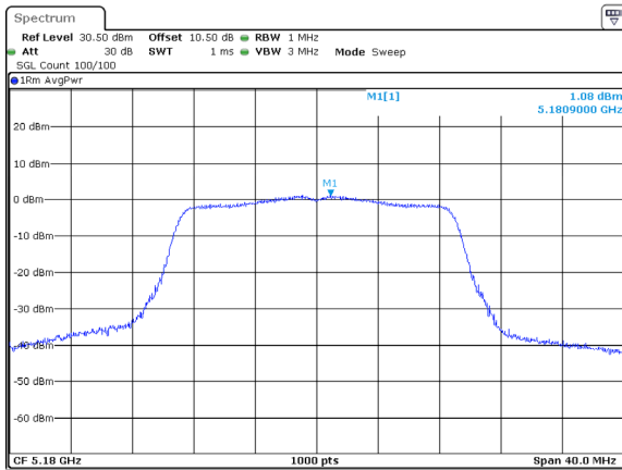
802.11ac20_5180MHz_ANT1
