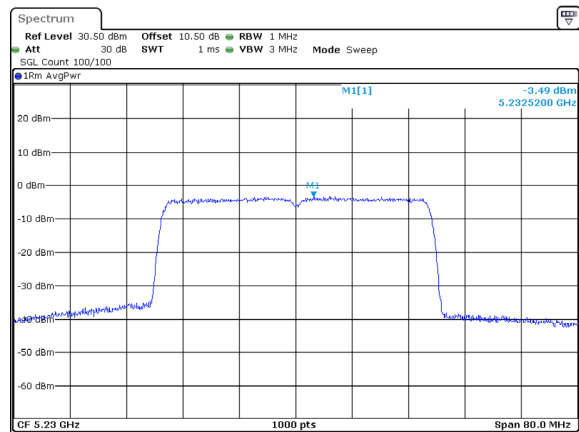
802.11ax40_5230MHz_RU_Full_ANT2
