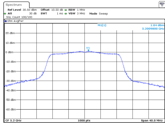
802.11ac20_5200MHz_ANT1
