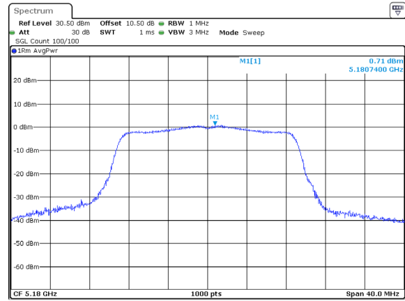
802.11ac20_5180MHz_ANT2
