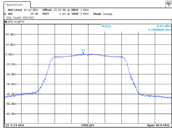
802.11ac20_5240MHz_ANT2
