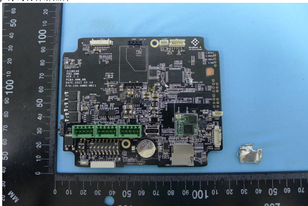
(26) 待測物拆解照片
