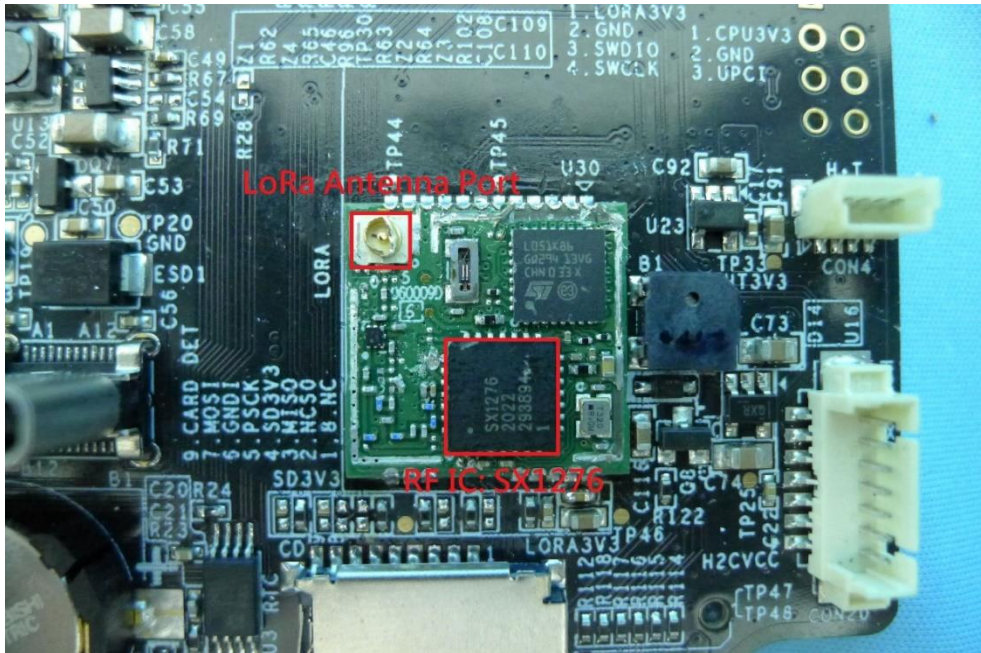
(28) 待測物拆解照片
