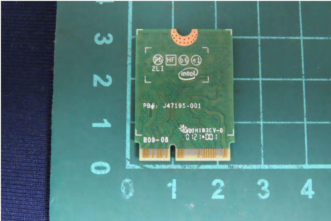
(7) EUT Photo_9560NGW
