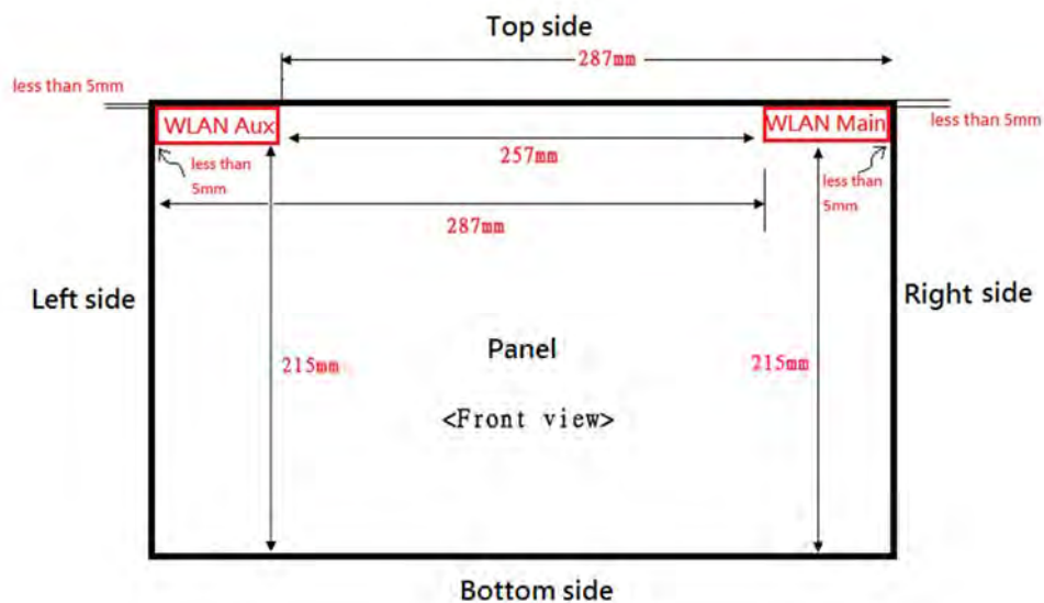
Fig.10 EUT (Laptop Mode)
