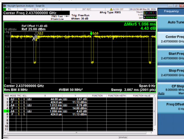
802.11ax-20 MHz(SU)
