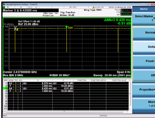
802.11b
