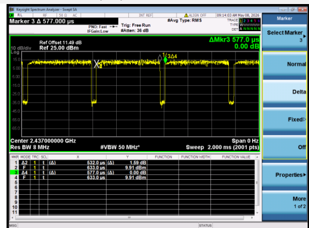
802.11ax-40 MHz(SU)
