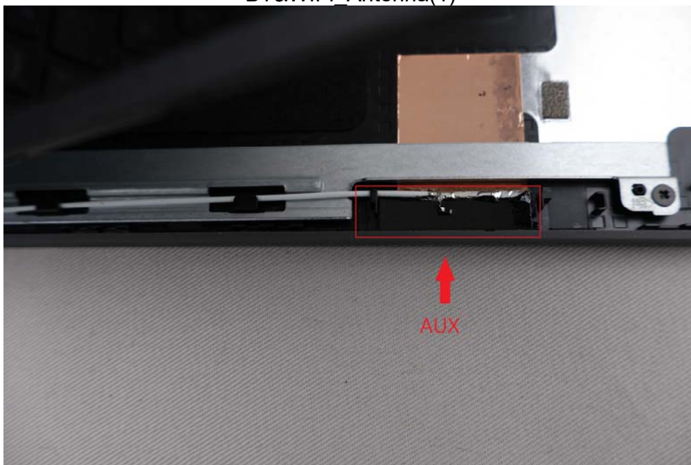
BT&WIFI_Antenna(1)
