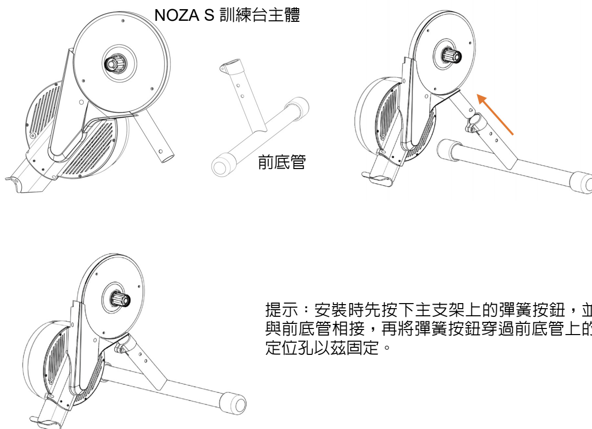
前底管安裝完成示意圖
