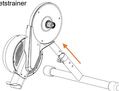
Voorste voet
