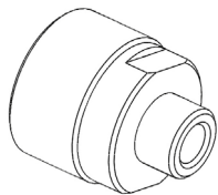
Adapter A - für Schnellspanner Kassettenmutter
