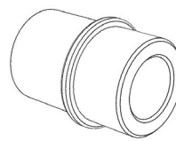
Adaptador D - Lado izquierdo para eje pesante de 12x142/ 12x148mm
