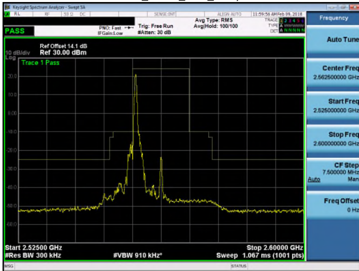
Band 7_QPSK_15M_RB1,74
