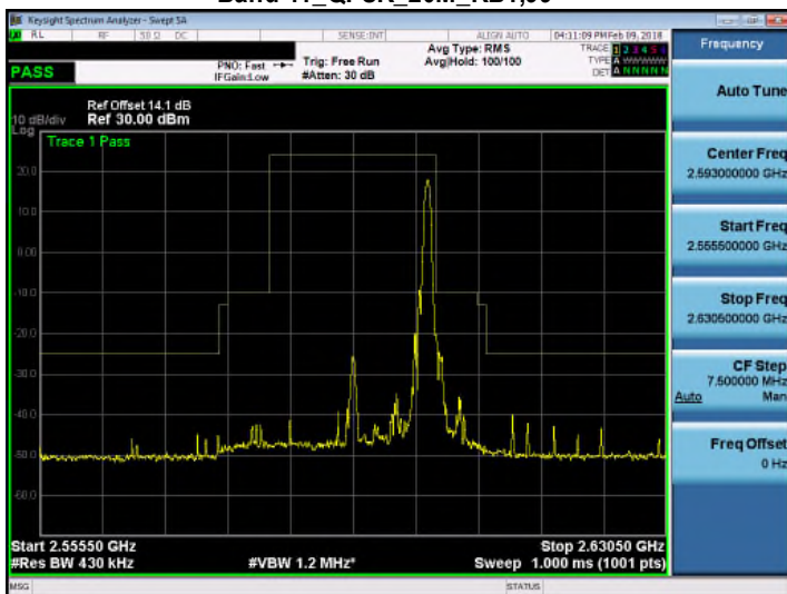
Band 41_QPSK_20M_RB1,99
