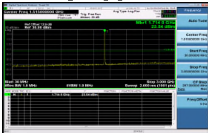
30MHz~3GHz_WCDMA_B4_LowCH1312-1712.4
