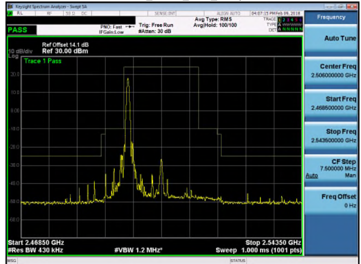
Band 41_QPSK_20M_RB1,99
