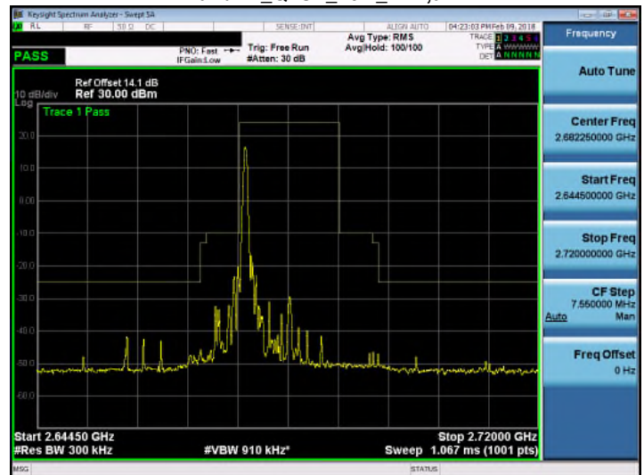
Band 41_QPSK_15M_RB1,74
