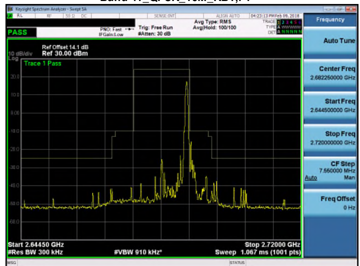
Band 41_QPSK_15M_RB1,74
