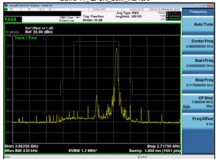
Band 41_QPSK_20M_RB1,99
