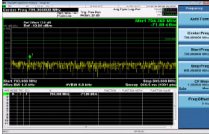
793MHz~805MHz Band13 5MHz QPSK 1_0 MidCH23230-782
