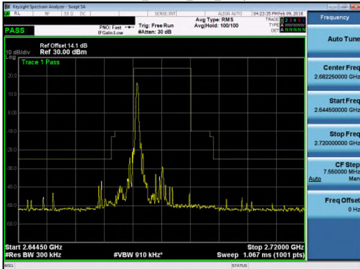
Band 41_16QAM_15M_RB1,74
