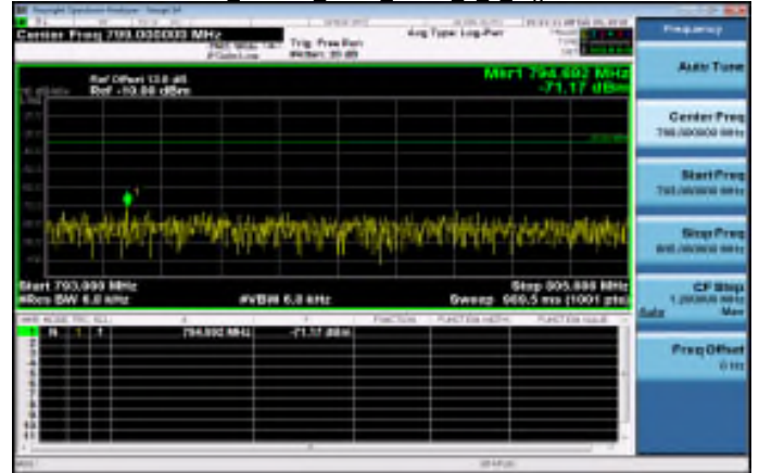
793MHz~805MHz Band13 5MHz QPSK 1_0 HighCH23255-784.5
