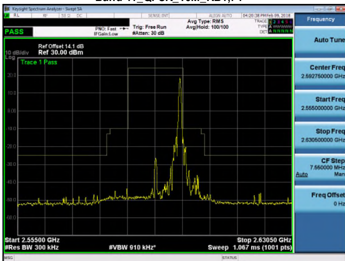
Band 41_QPSK_15M_RB1,74
