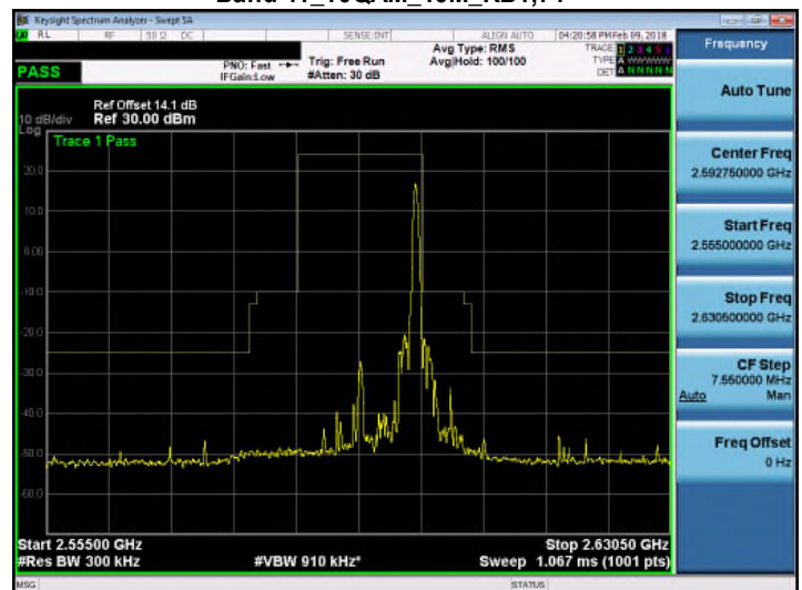
Band 41_16QAM_15M_RB1,74
