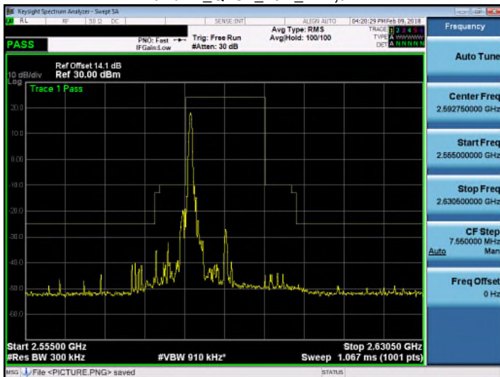
Band 41_QPSK_15M_RB1,74
